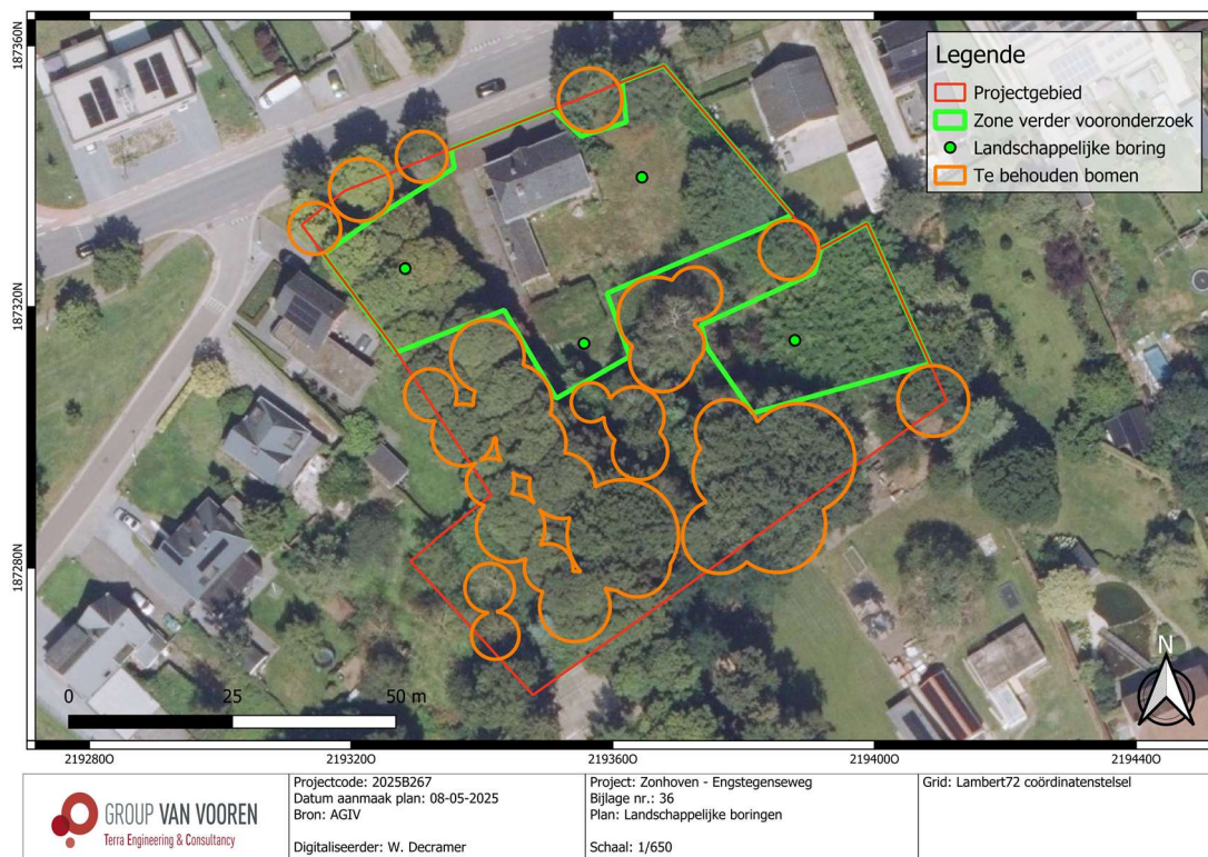
Fig. 2.7: Voorstel boorpuntenplan op de meest recente luchtfoto (2023) (© AGIV).
