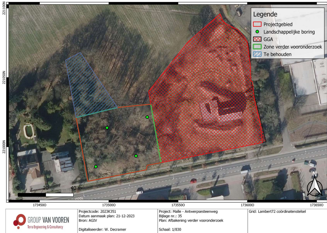
Fig. 2.6: Voorstel boorpuntenplan.
