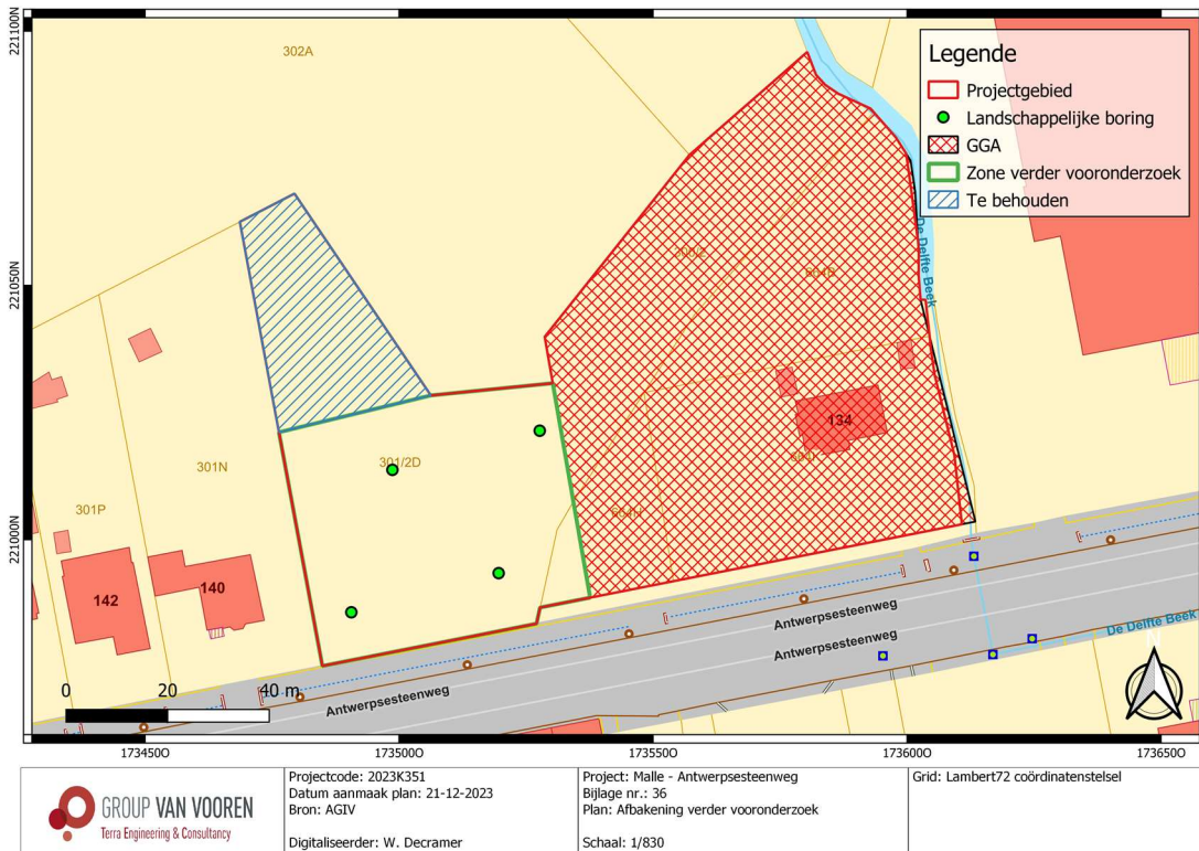
Fig. 2.7: Voorstel boorpuntenplan.
