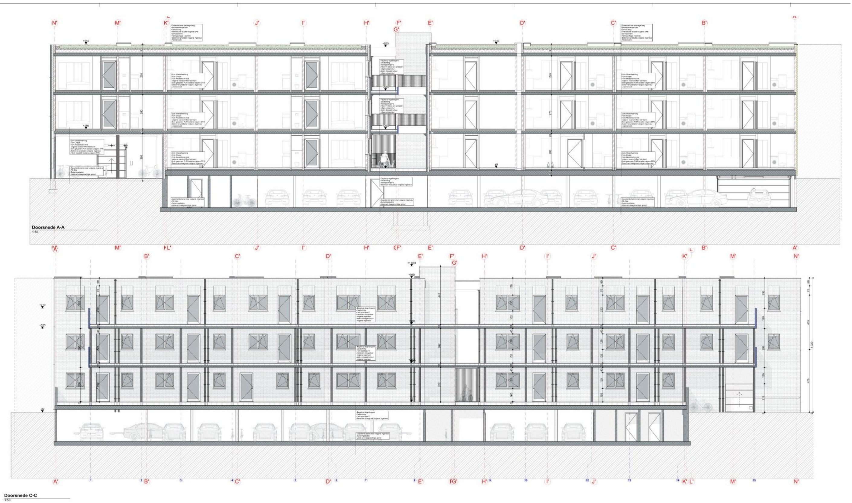
Figuur 7: Langsdoorsneden ontworpen toestand (Atrium Architecten)
