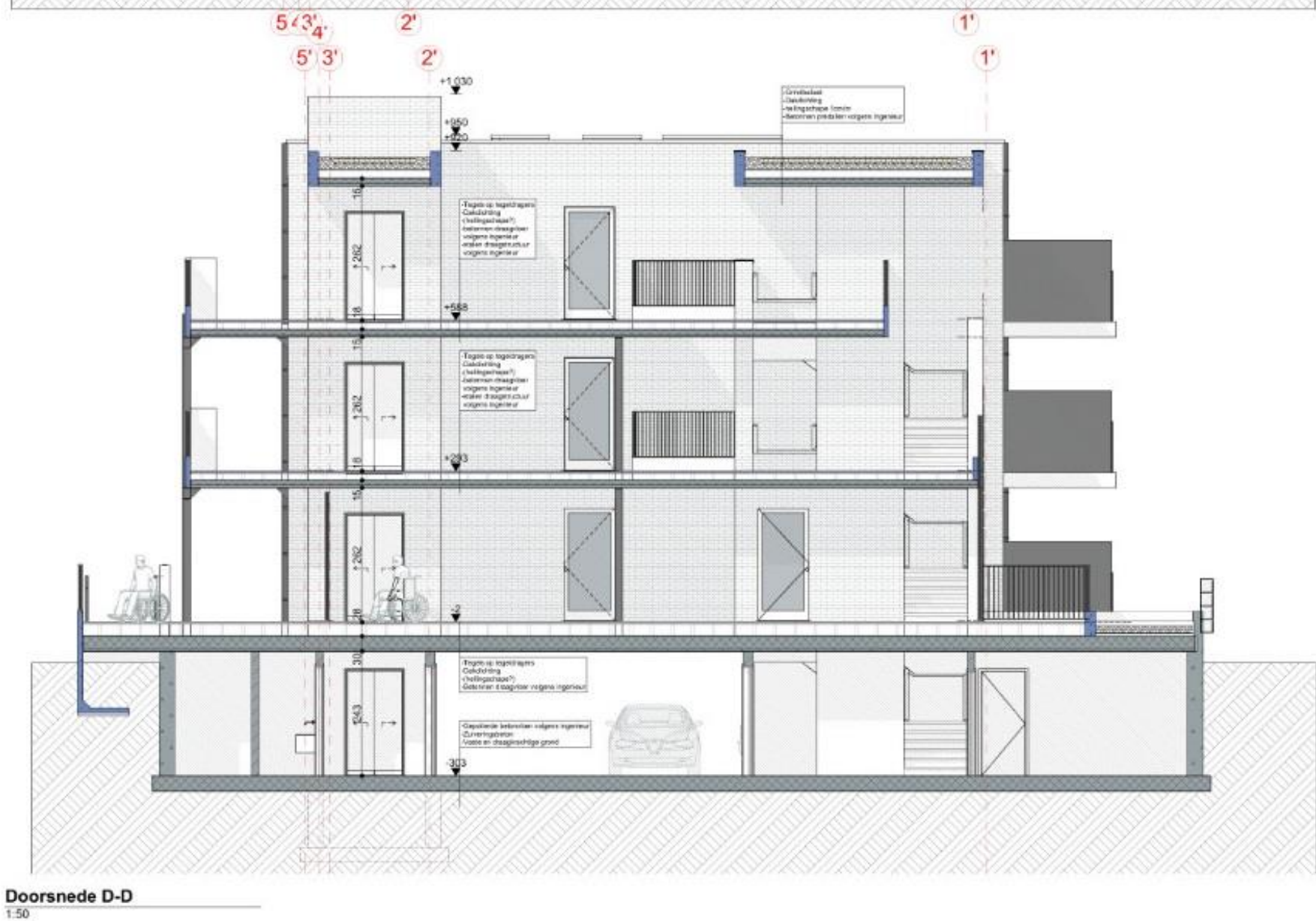
Figuur 8: Dwarsdoorsneden ontworpen toestand (Atrium Architecten)
