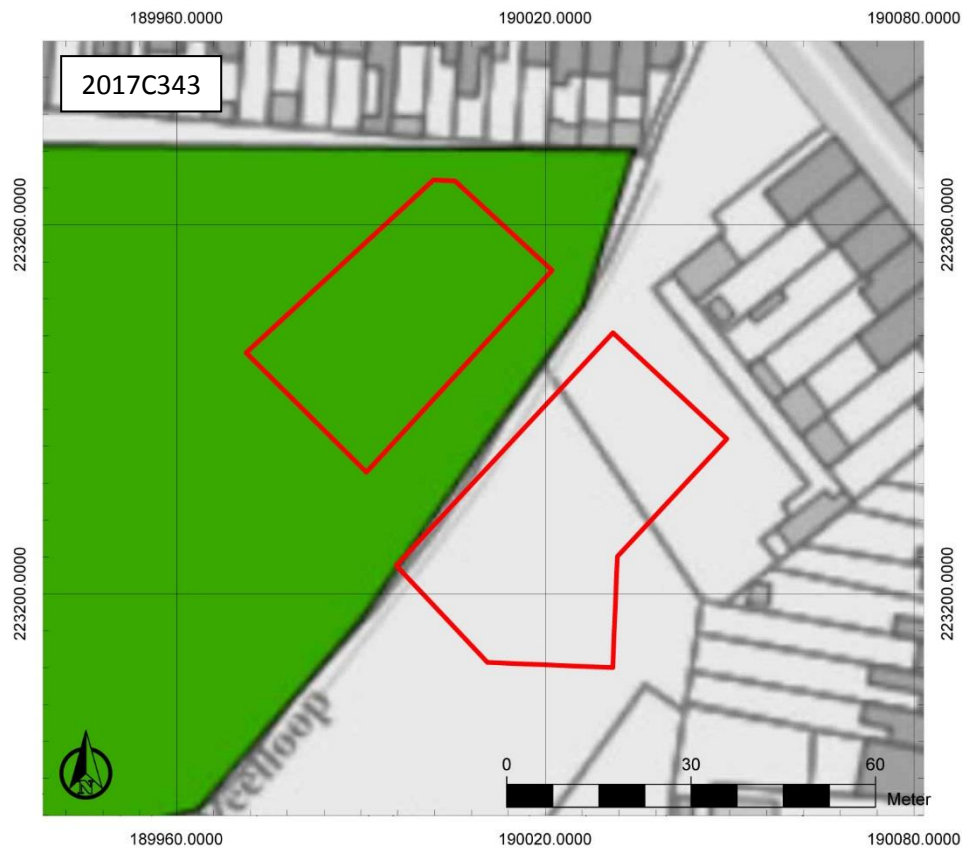
Figuur 18: Potentiële bodemerosiekaart met aanduiding van het onderzoeksgebied ( www.geopunt.be )
