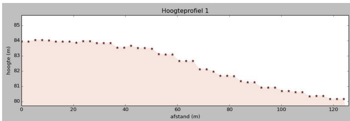
Figuur 12: Hoogteprofiel 1: zuidwest-noordoost (bron: Geopunt).
