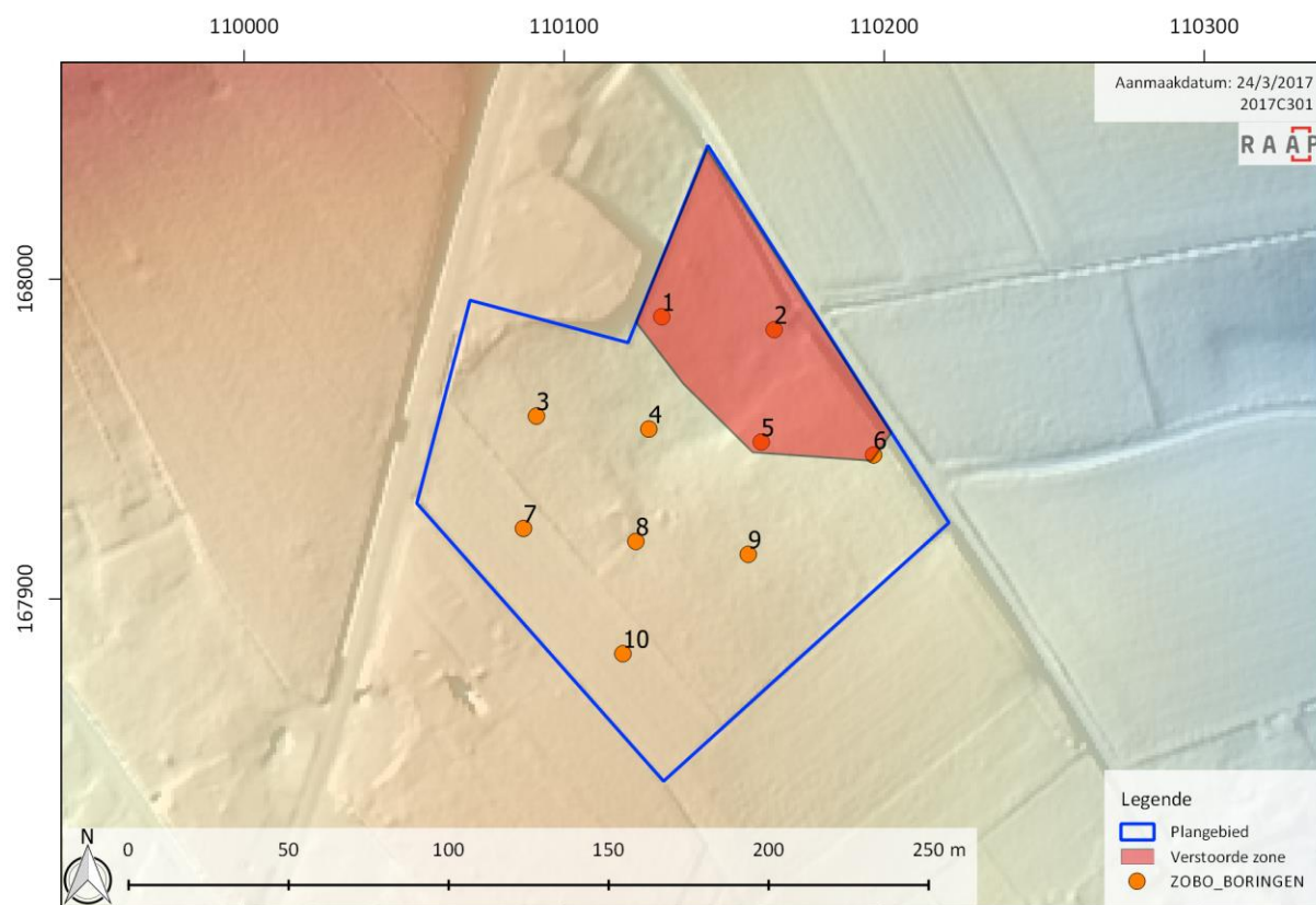
Figuur 33: Plangebied weergegeven op het DTM met aanduiding van de verstoorde zone (bron: AGIV).
