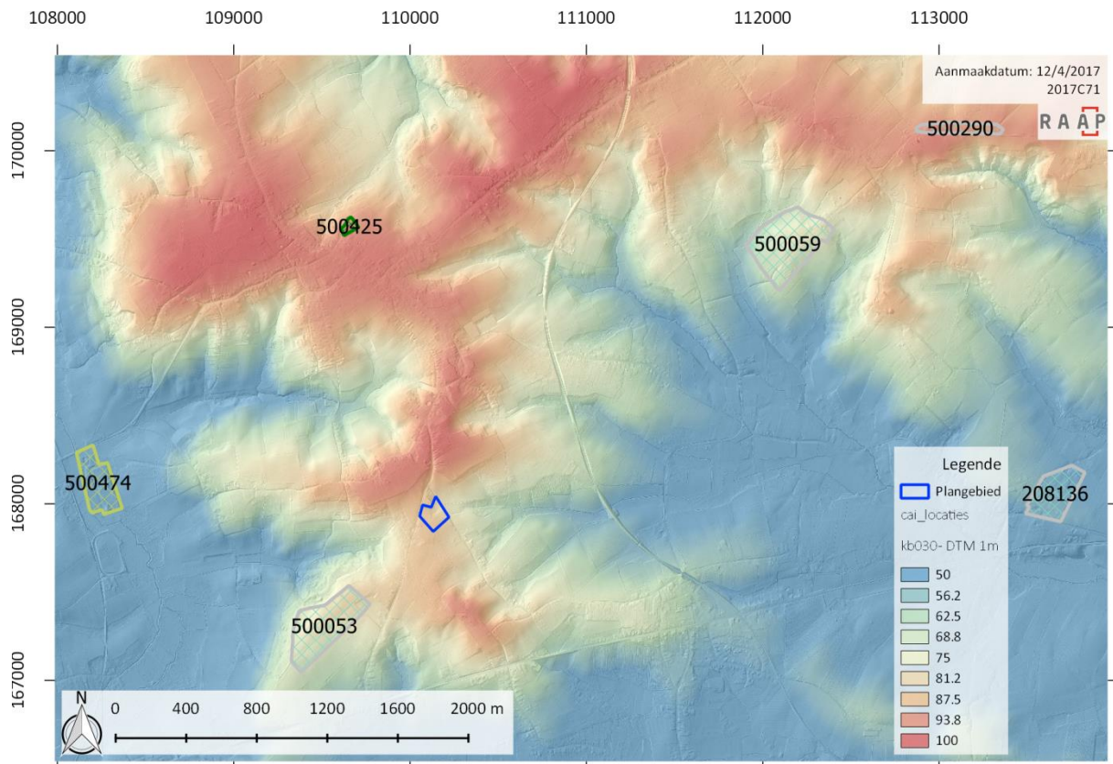
Figuur 16: Plangebied weergegeven op DTM en shadowmap met aanduiding van CAI polygonen (bron: Onroerend Erfgoed, AGIV).
