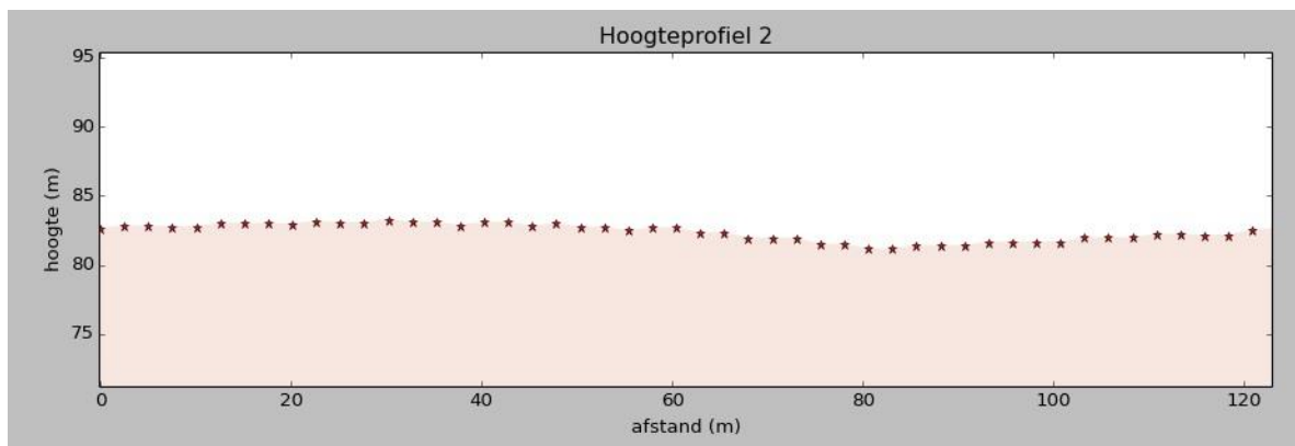
Figuur 13: Hoogteprofiel 2: noordwest-zuidoost (bron Geopunt).
