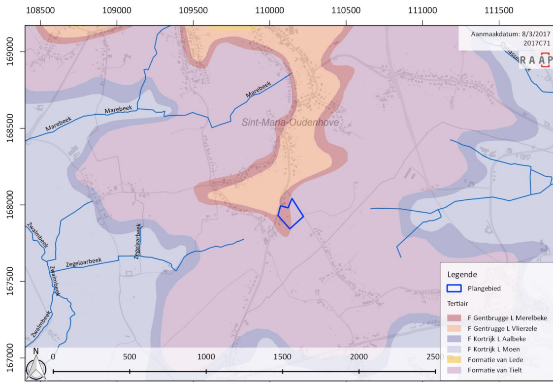
Figuur 7: Tertiair geologische kaart met aanduiding van het plangebied en de waterlopen in de omgeving (bron: DOV, Grootschalig Referentiebestand Vlaanderen, AGIV, VMM).
