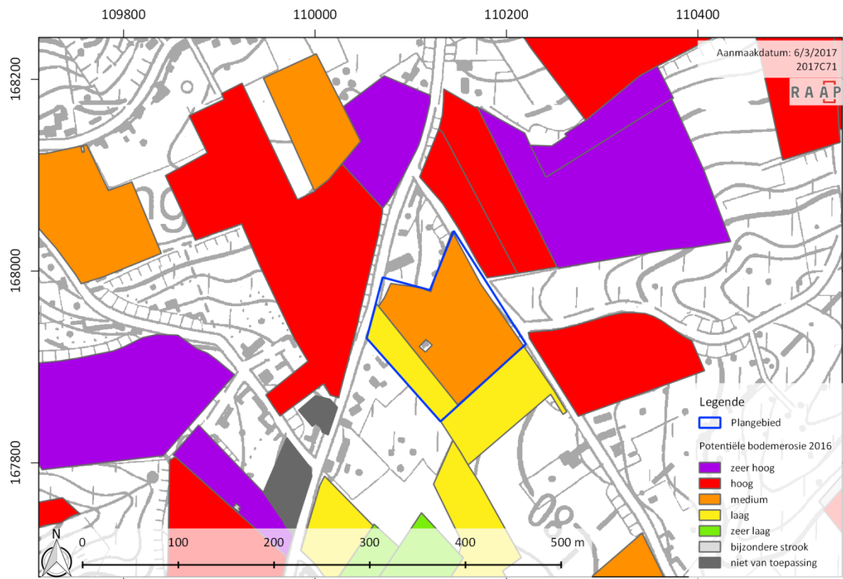
Figuur 15: Potentiële bodemerosiekaart uit 2016 (bron: DOV, Grootchalig Referentiebestand Vlaanderen, AGIV).
