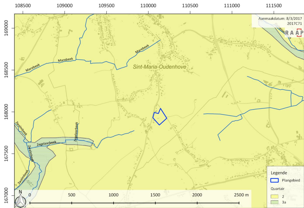
Figuur 8: Quartair geologische kaart geprojecteerd op de GRB-kaart. (bron: DOV, Grootchalig Referentiebestand Vlaanderen, AGIV).
