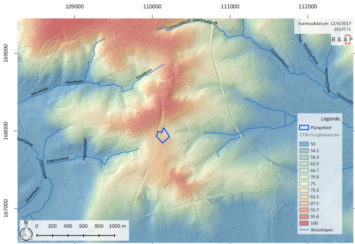
Figuur 10: Digitaal Terreinmodel Vlaanderen met shadowmap en aanduiding van het plangebied en waterlopen (bron: AGIV & VMM).
