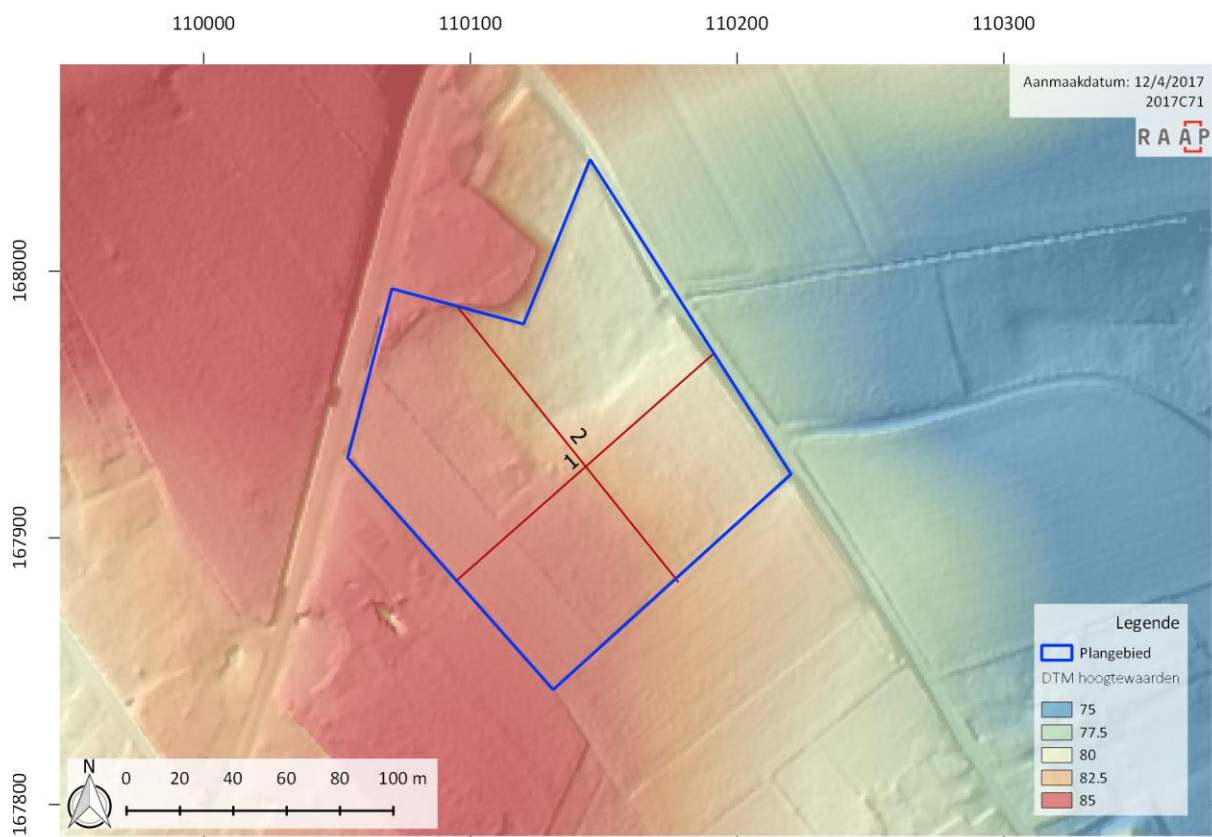
Figuur 11: Plangebied op hoogtemodel met aanduiding van hoogteprofielen (bron: Geopunt & AGIV).
