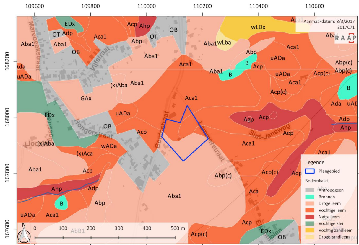
Figuur 9: Bodemkaart met projectie van het plangebied (bron: DOV, Grootschalig Referentiebestand Vlaanderen, AGIV).
