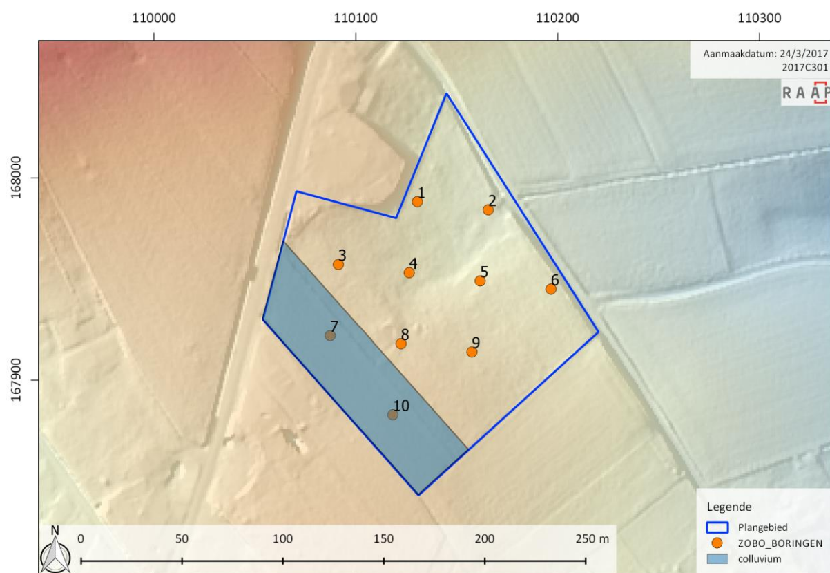
Figuur 34: Plangebied weergegeven op het DTM met aanduiding van het colluvium (bron: AGIV).
