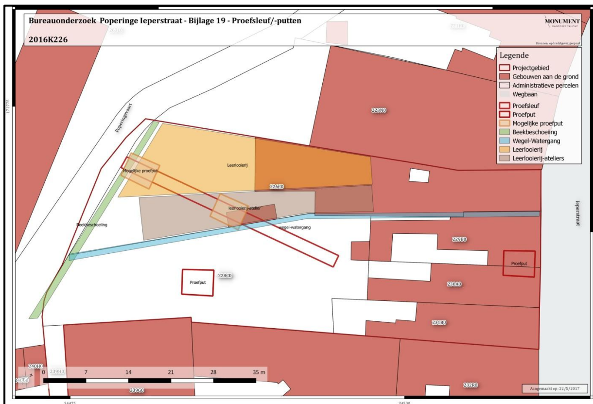
Figuur 2: Overzichtsplan met inplanting van de proefsleuf/-put.
