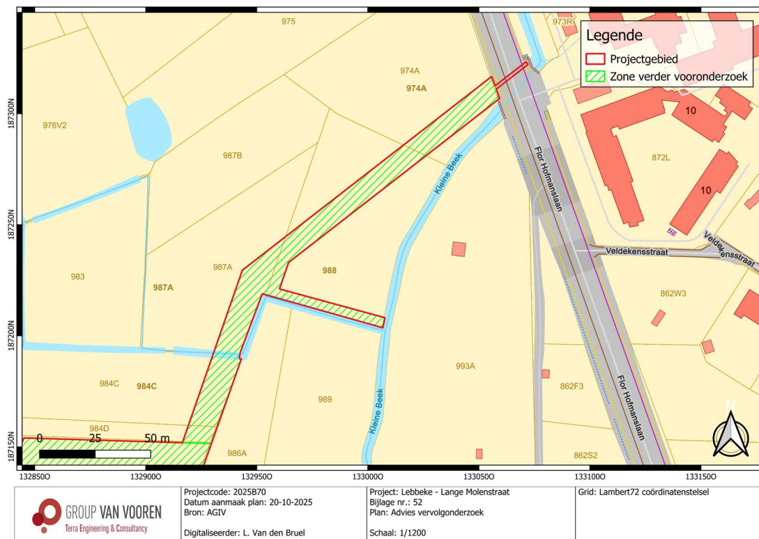
Fig. 2.10: Zone advies vervolgonderzoek ter hoogte van de zone met de geplande DWA-leiding geprojecteerd op het kadasterplan (@ AGIV).
