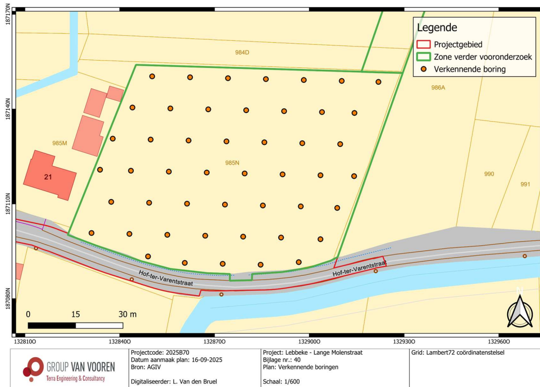
Fig. 2.14: Voorstel verkennende archeologische boringen op het kadasterplan (© AGIV).
