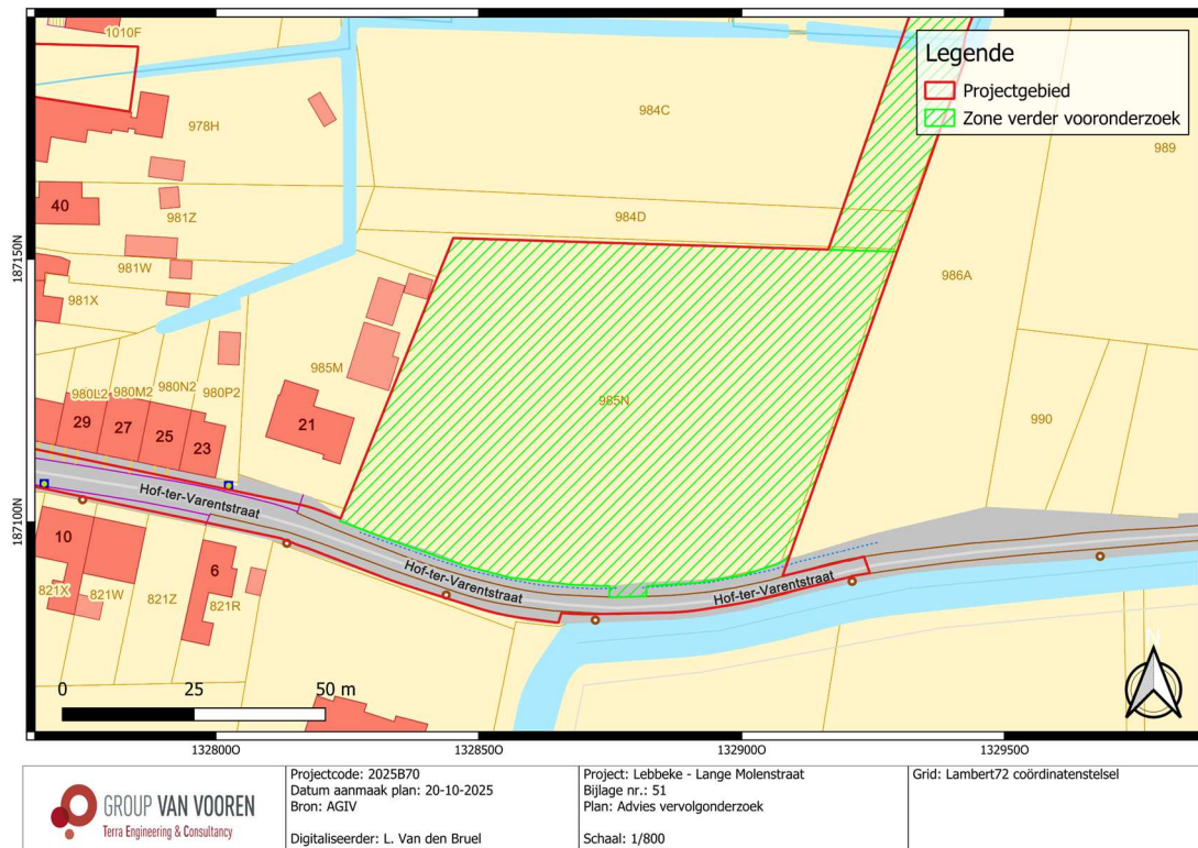
Fig. 2.8: Zone advies vervolgonderzoek ter hoogte van de grondverbeteringszone geprojecteerd op het kadasterplan (© AGIV).
