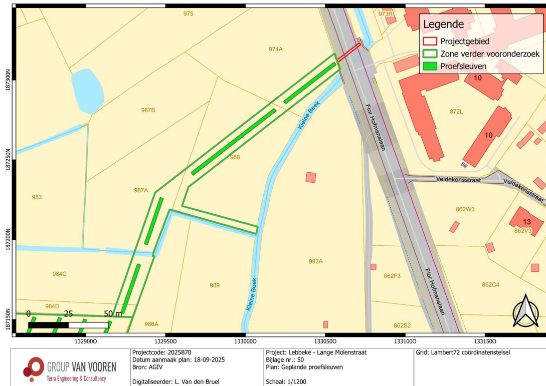
Fig. 2.22: Voorstel inplanting proefsleuven op het kadasterplan (© AGIV).
