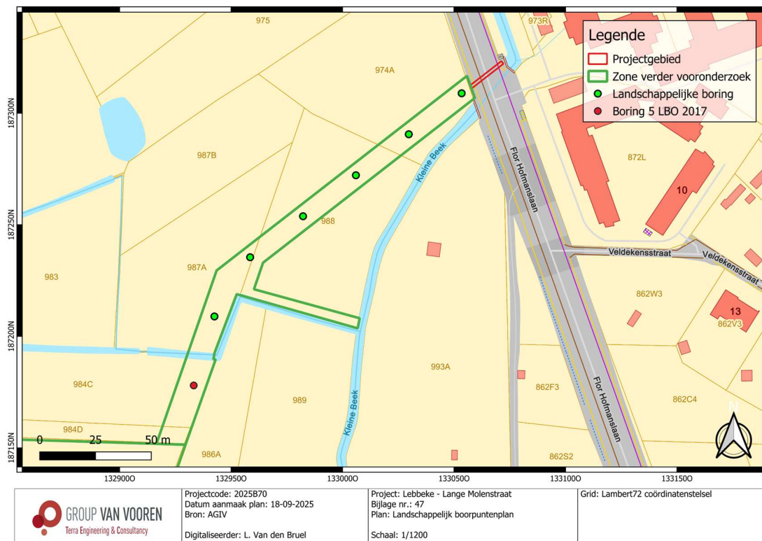
Fig. 2.19: Voorstel boorpuntenplan op het kadasterplan (@ AGIV).
