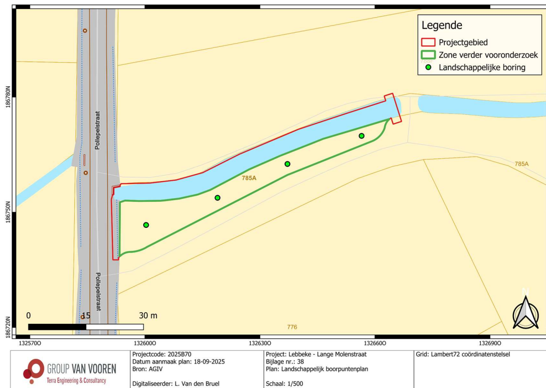
Fig. 2.25: Voorstel boorpuntenplan op het kadasterplan (@ AGIV).
