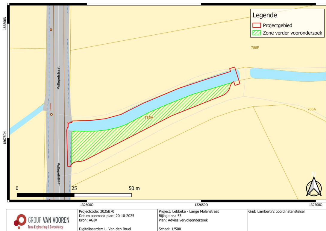
Fig. 2.12: Zone advies vervolgonderzoek ter hoogte van het bufferbekken geprojecteerd op het kadasterplan (© AGIV).
