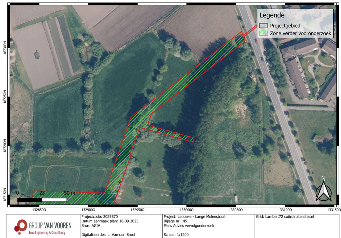
Fig. 2.9: Zone advies vervolgonderzoek ter hoogte van de zone met de geplande DWA-leiding geprojecteerd op de meest recente luchtfoto (2023) (@ AGIV).
