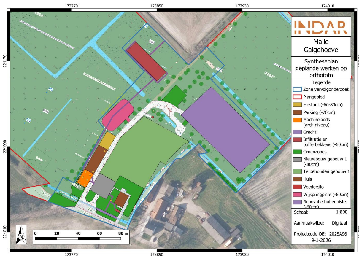
Figuur 4: Plangebied met synthese geplande werken op orthofoto.
