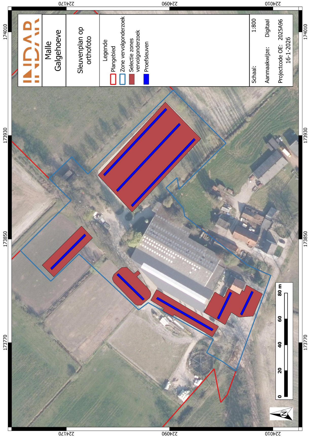
Figuur 6: Sleuvenplan op orthofoto.
