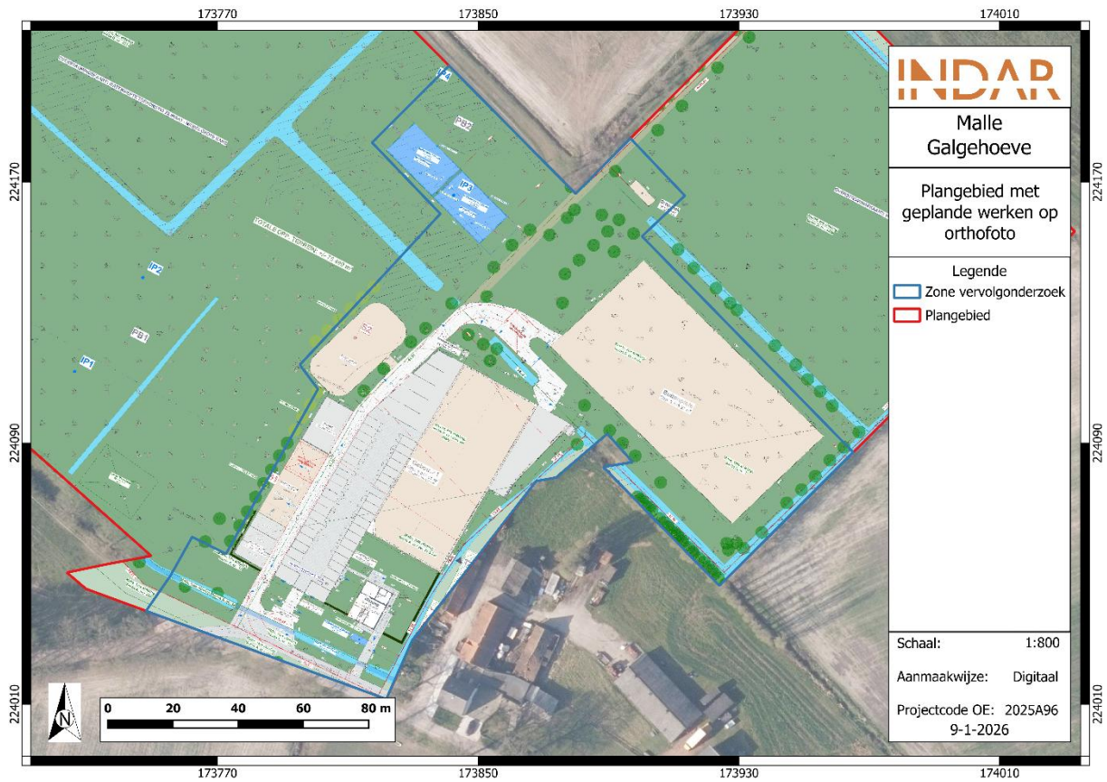
Figuur 3: Plangebied met weergave van toekomstige inplanting 4 op orthofoto.
