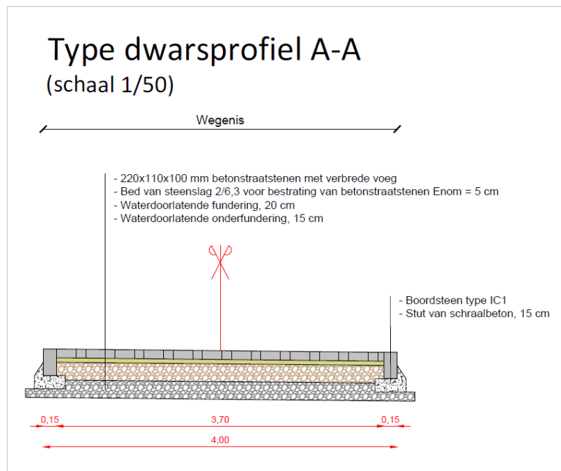
Figuur 2: Dwarsprofiel wegnis (opdrachtgever, 2026)
