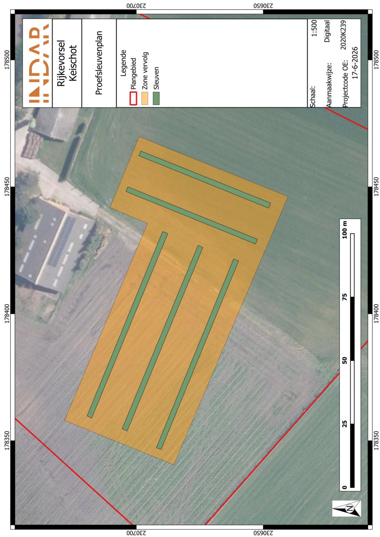
Figuur 4: Sleuvenplan
