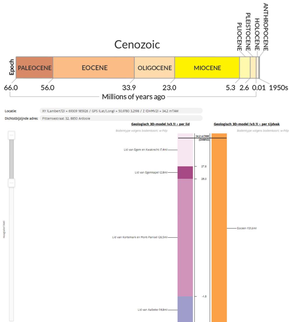
Figuur 22. Geologisch 3D-model van het onderzoeksgebied.
