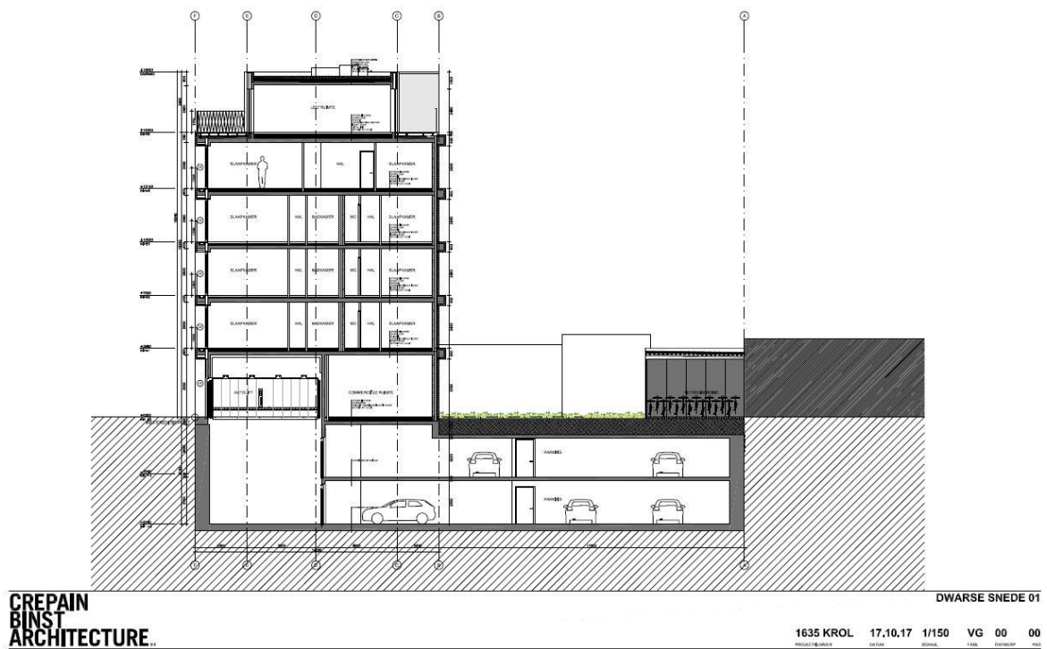
Figuur 3: Nieuwe inplanting doorsnede
