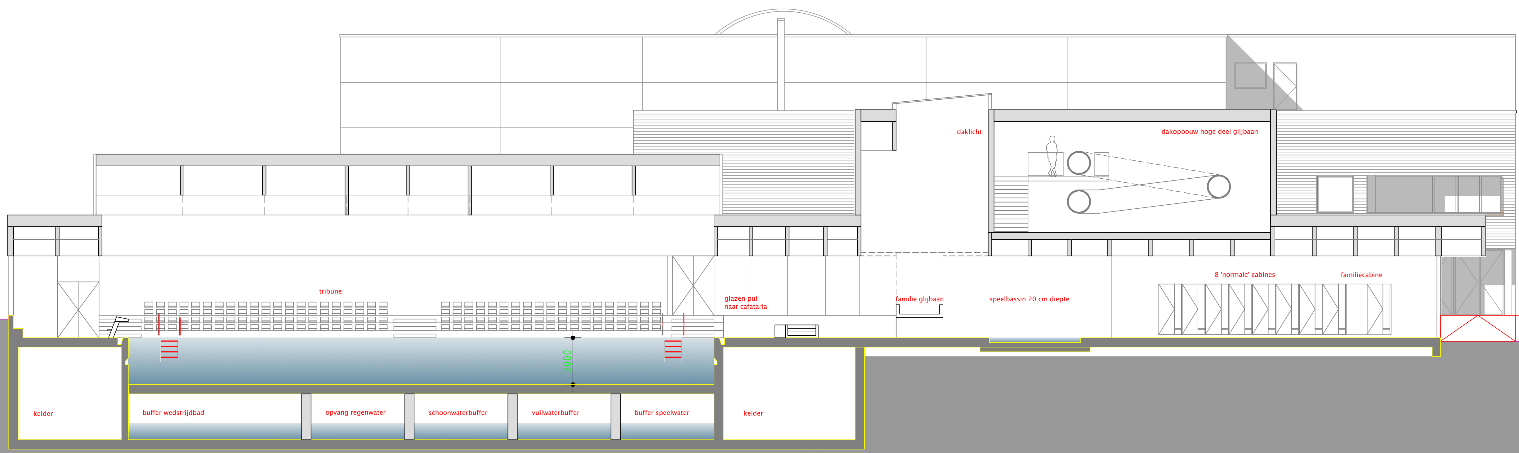
snede A
