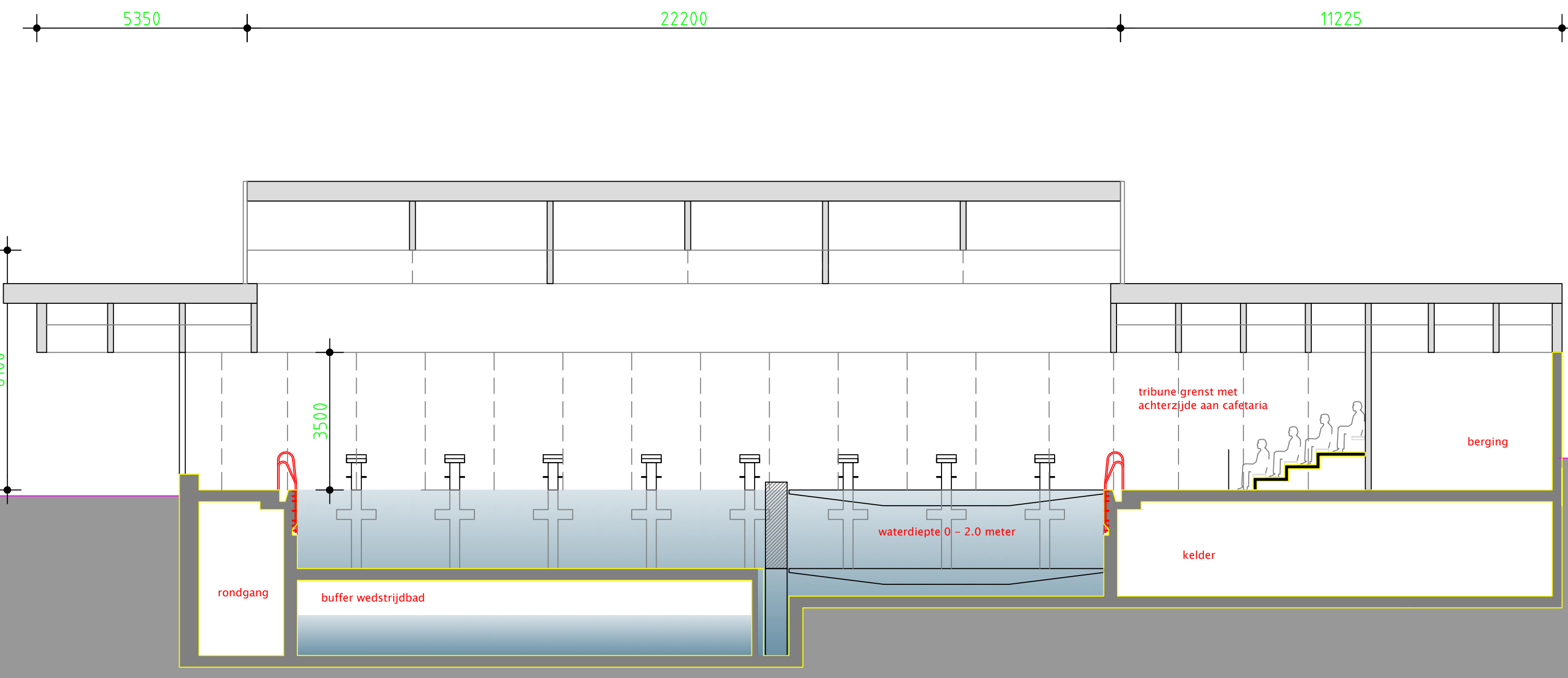
snede B
