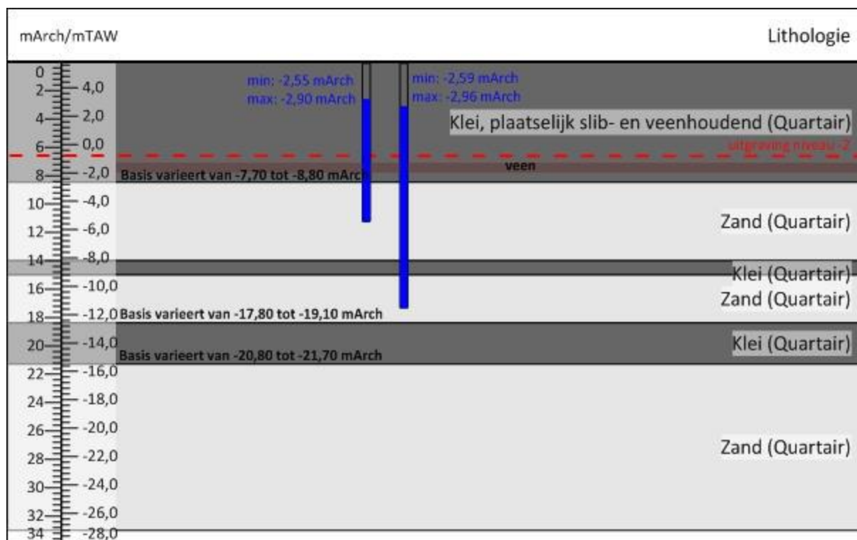
Figuur 12: Vereenvoudigd hydrogeologisch profiel (Bemalings- en zettingsadvies. Project Residentie Imperial te Oostende. Rapport AGT nv)
