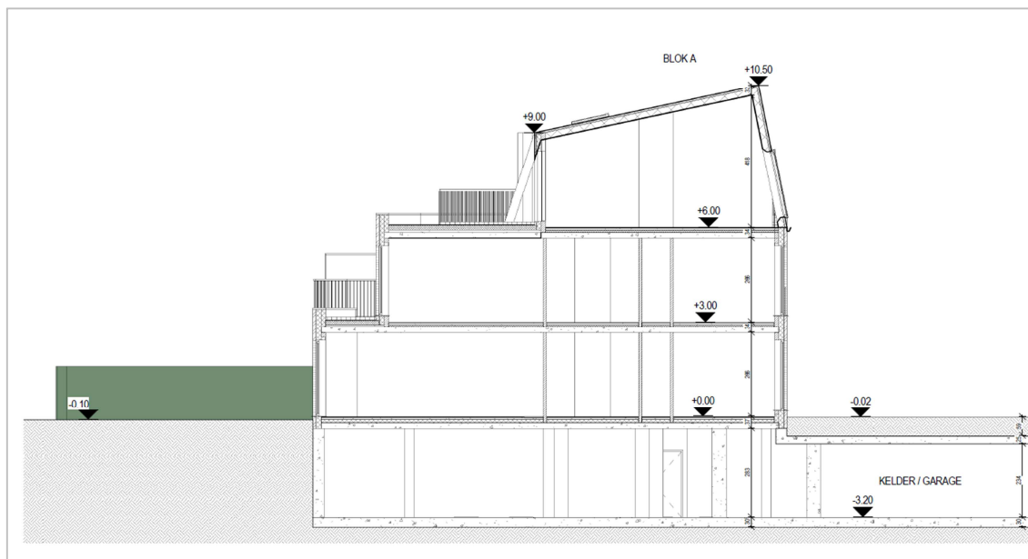
Figuur 3: Snede kelderverdieping (ABML, juni 2017)
