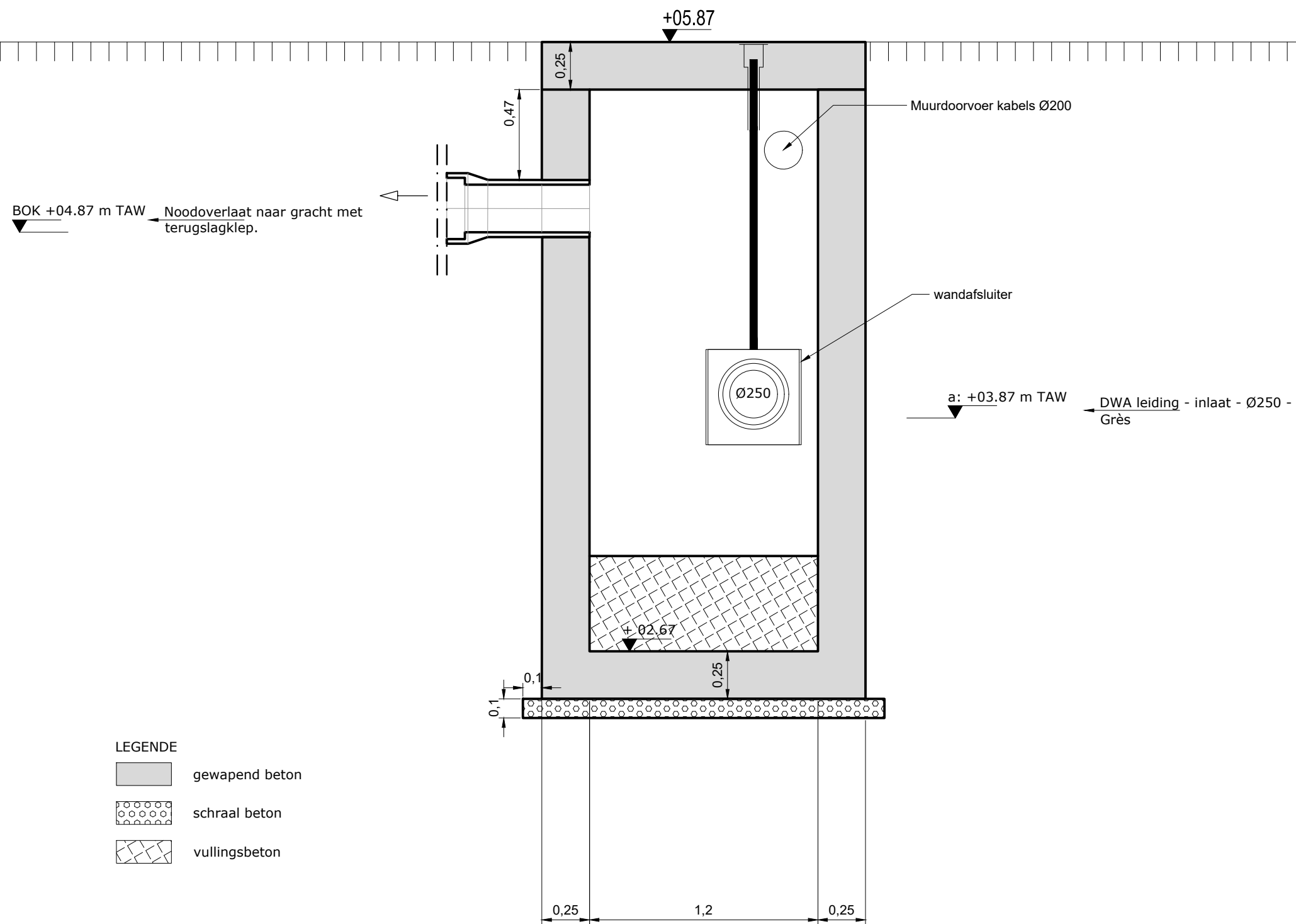
Detail pompstation - doorsnede B-B' schaal 1/ 25 - plan 06/06 c
