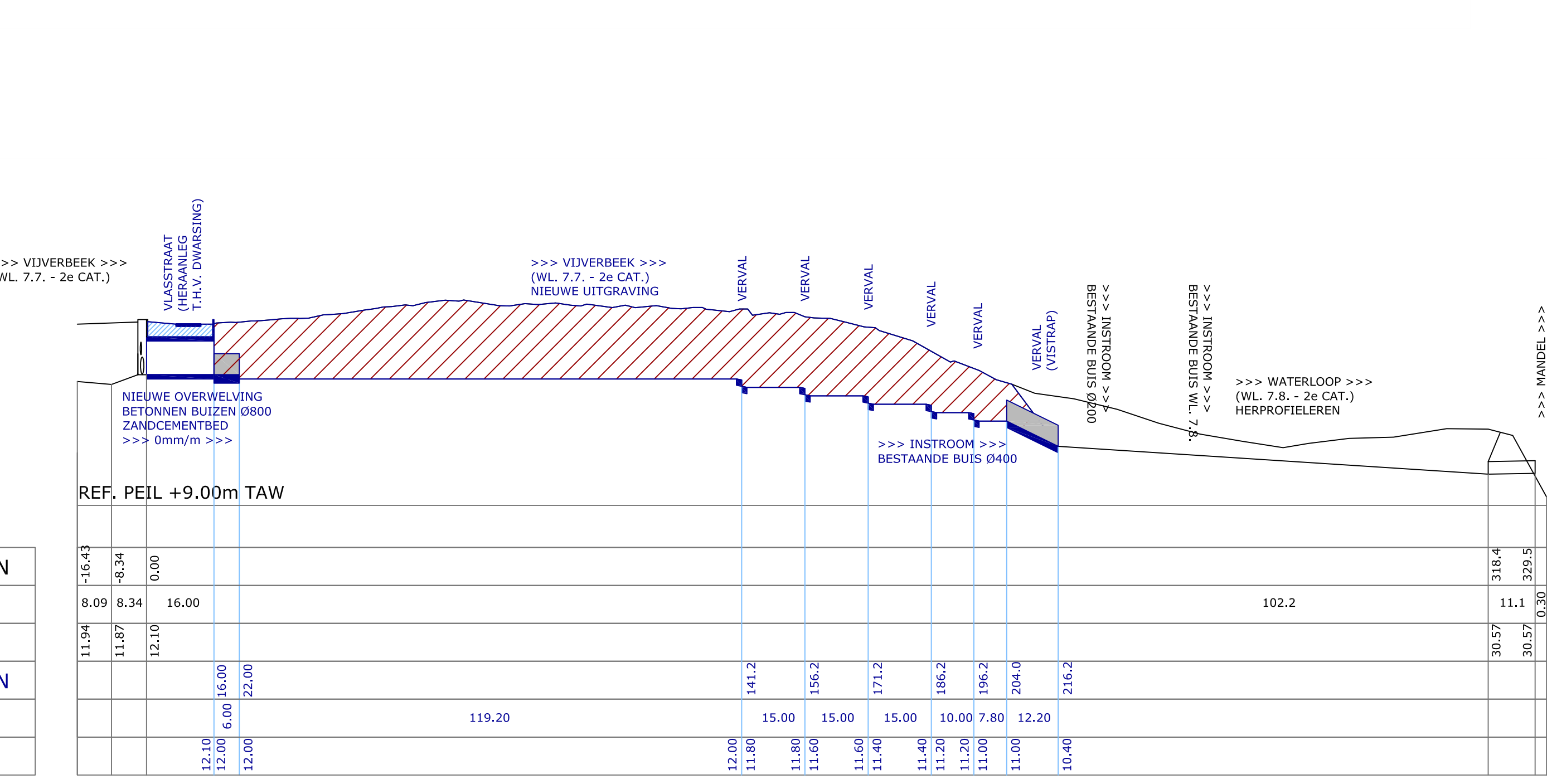
TYPEDWARSPROFIEL T.H.V. NIEUWE WEGGRACHT
