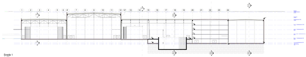
Afbeelding 3: Doorsnede van de toekomstige situatie van noord (links) naar zuid (rechts). Centraal is de locatie van het zwembad herkenbaar door de lokale verdieping in de ondergrond.
