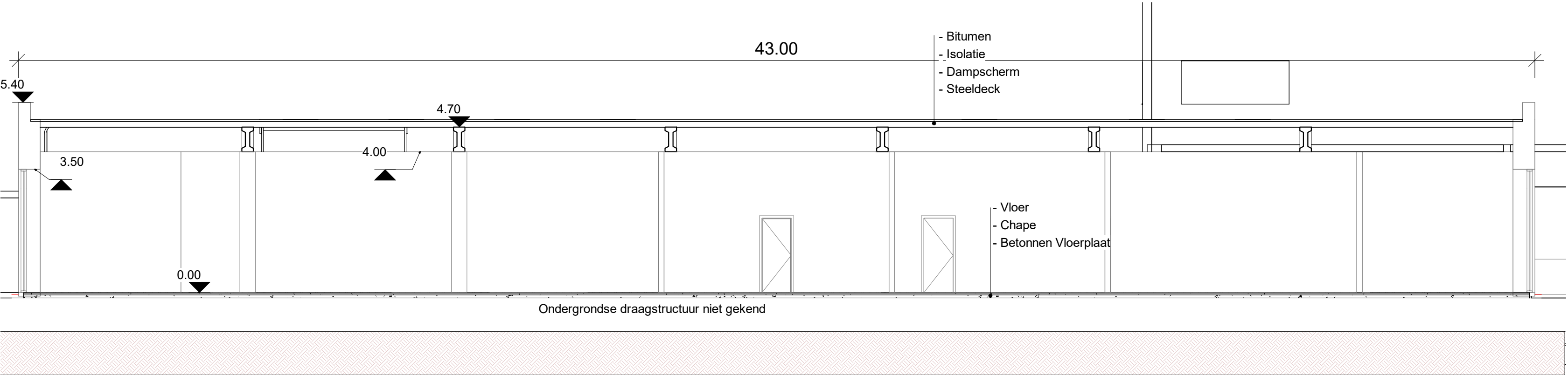
1 Langssnede bestaande kantoren 1: 100
