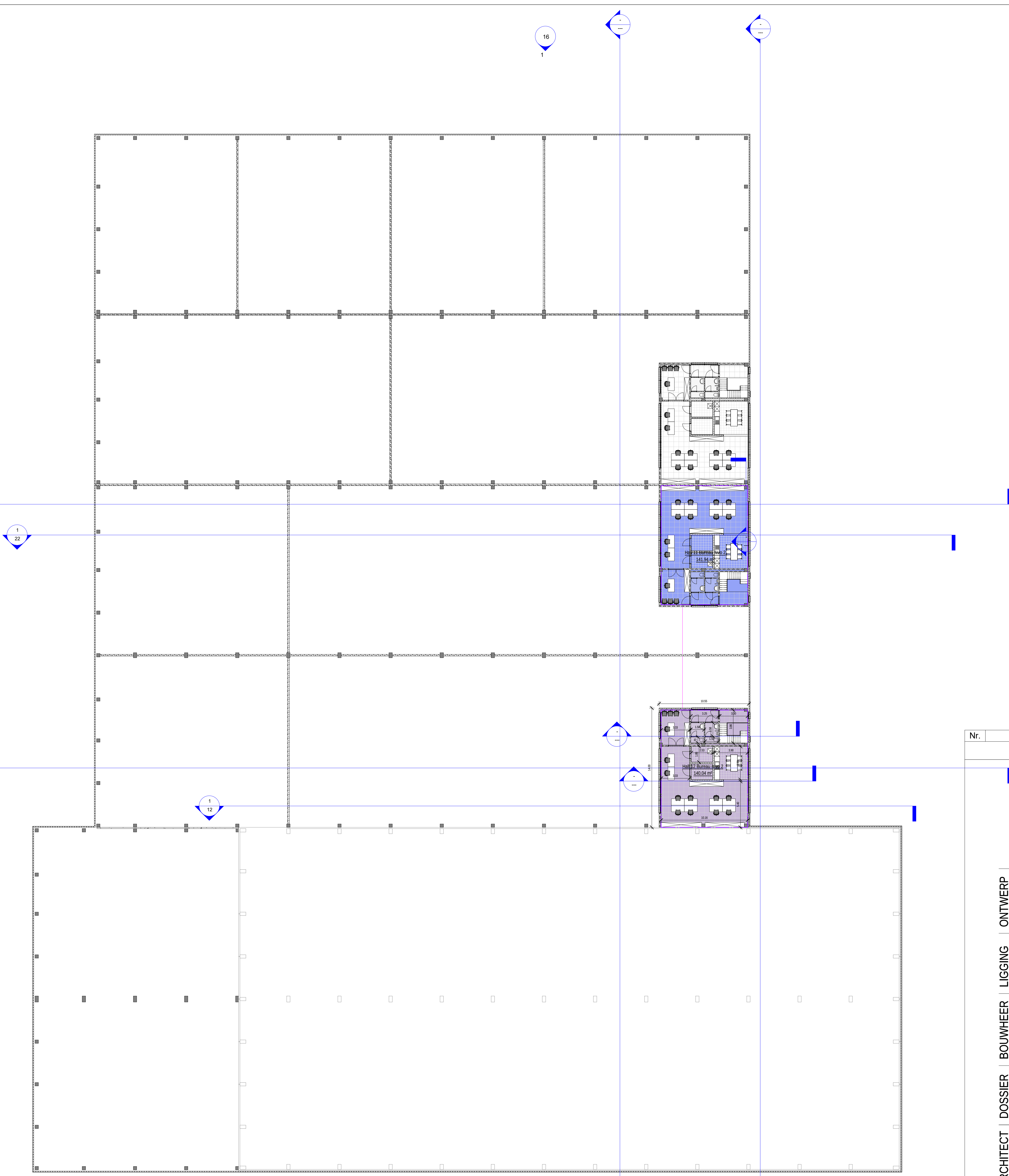
1 Bureau Hall 11 en 12 Verdieping 2 1:200
