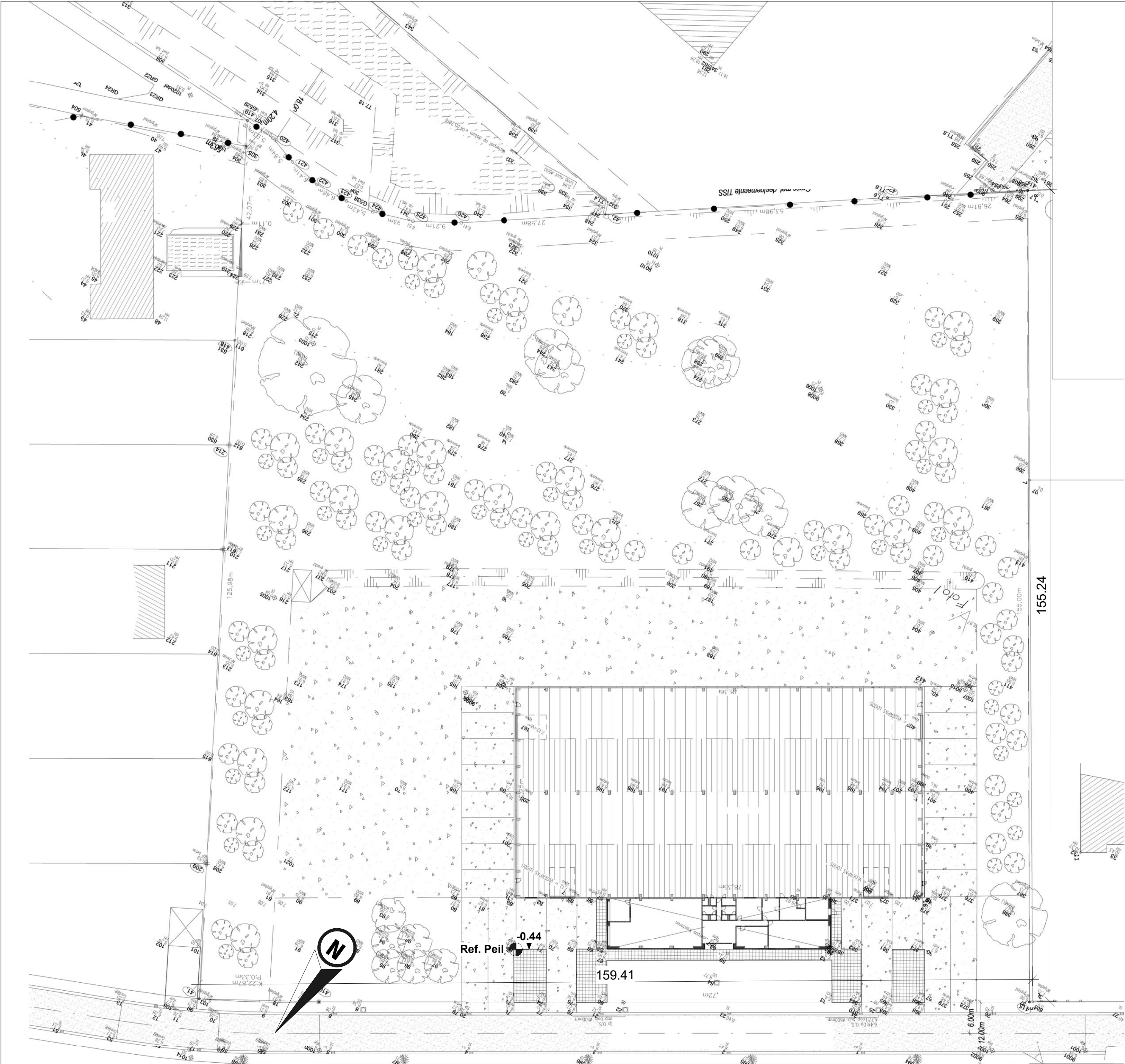
Bestaande Toestand Inplanting 1:500
