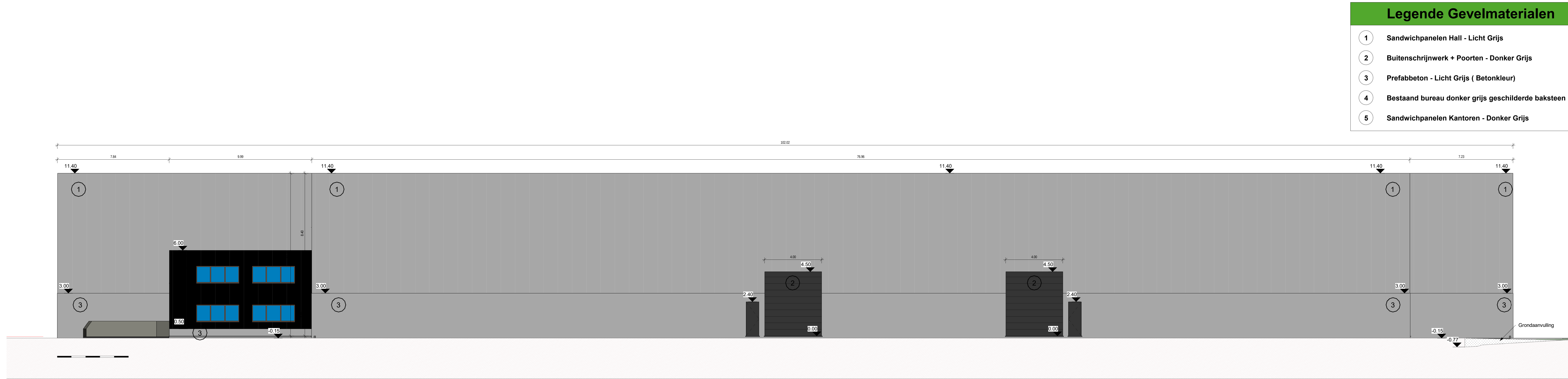
1 Achtergevel nieuwe toestand 1:100
