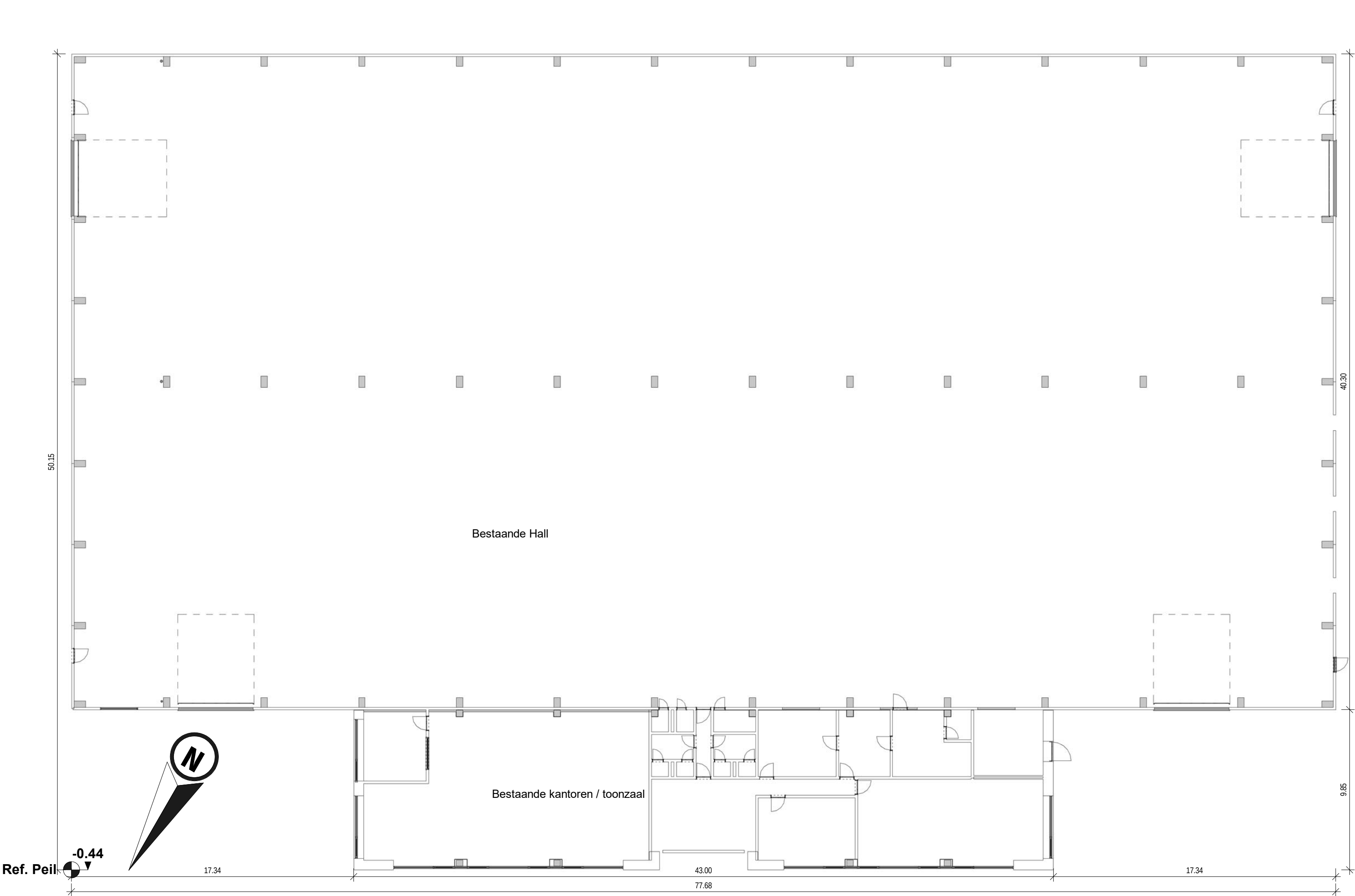
1 Bestaande Toestand Plan 1 : 200
