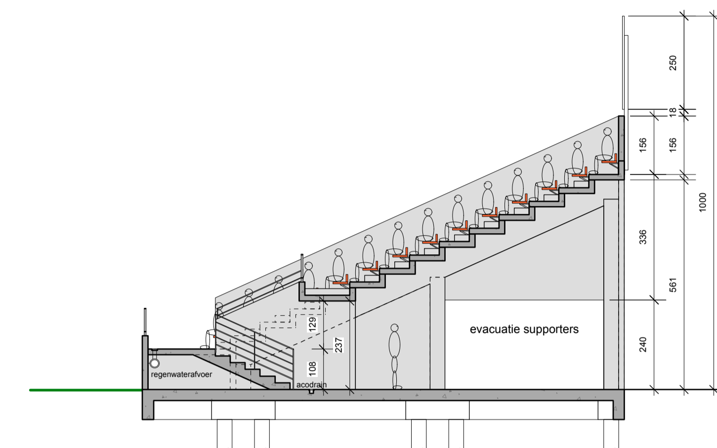
DOORSNEDE A - A'
