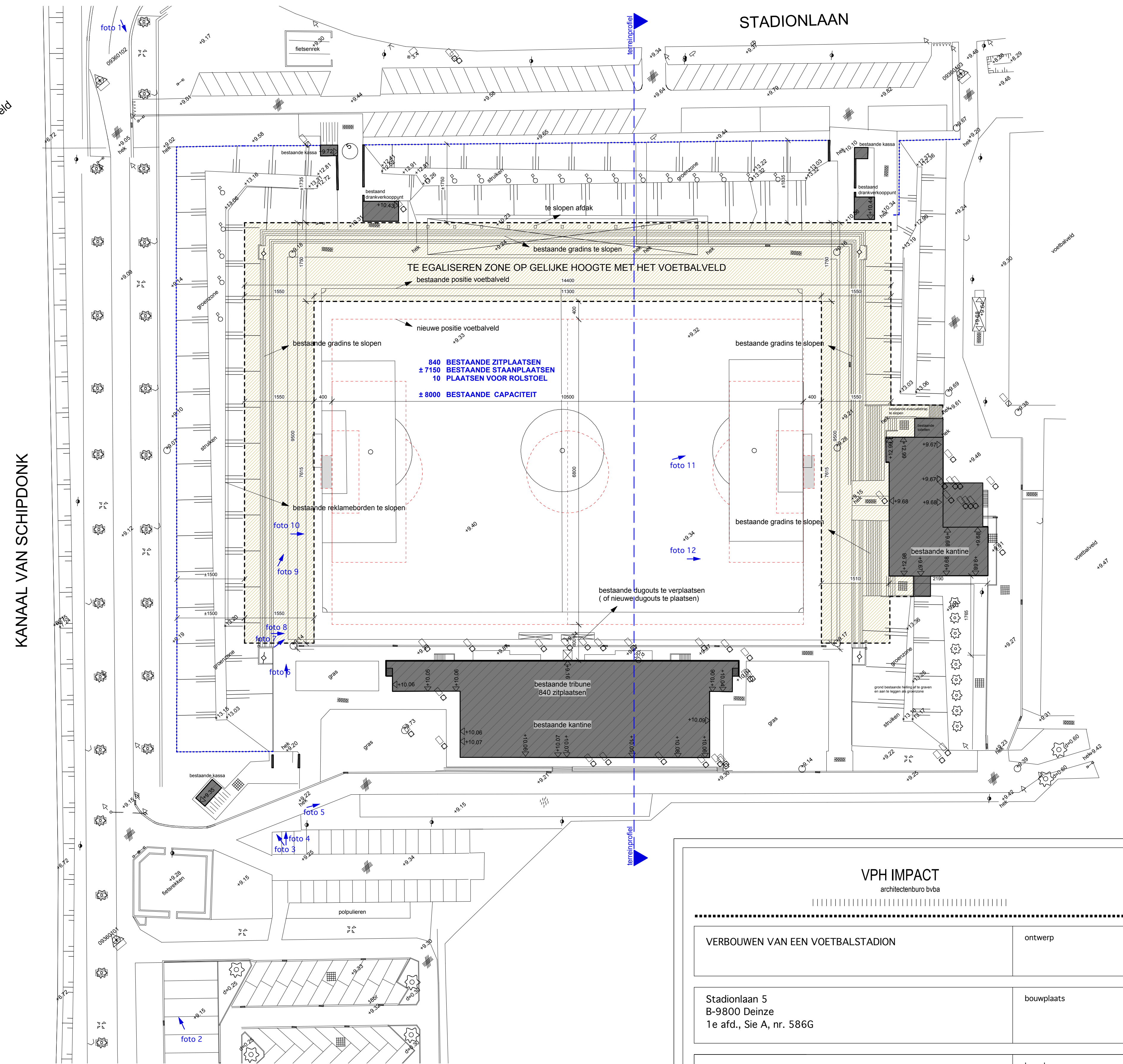
bestaande toestand INPLANTINGSPLAN
