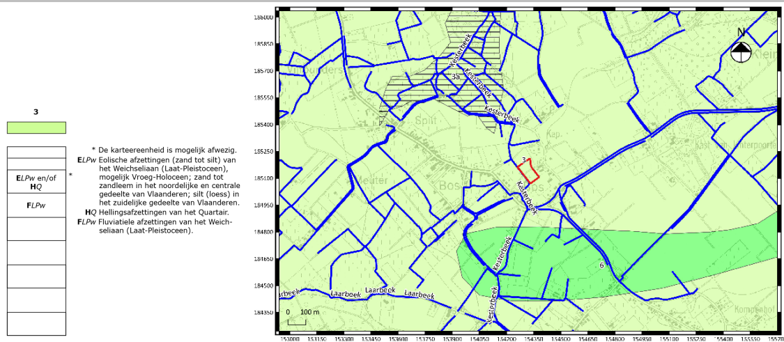
Fig. 1.10: Detail uit de quartair geologische kaart met aanduiding van het projectgebied.
