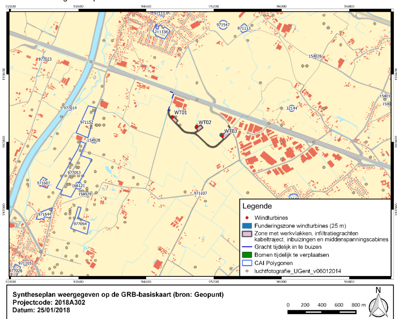
Figuur 26: syntheseplan.
