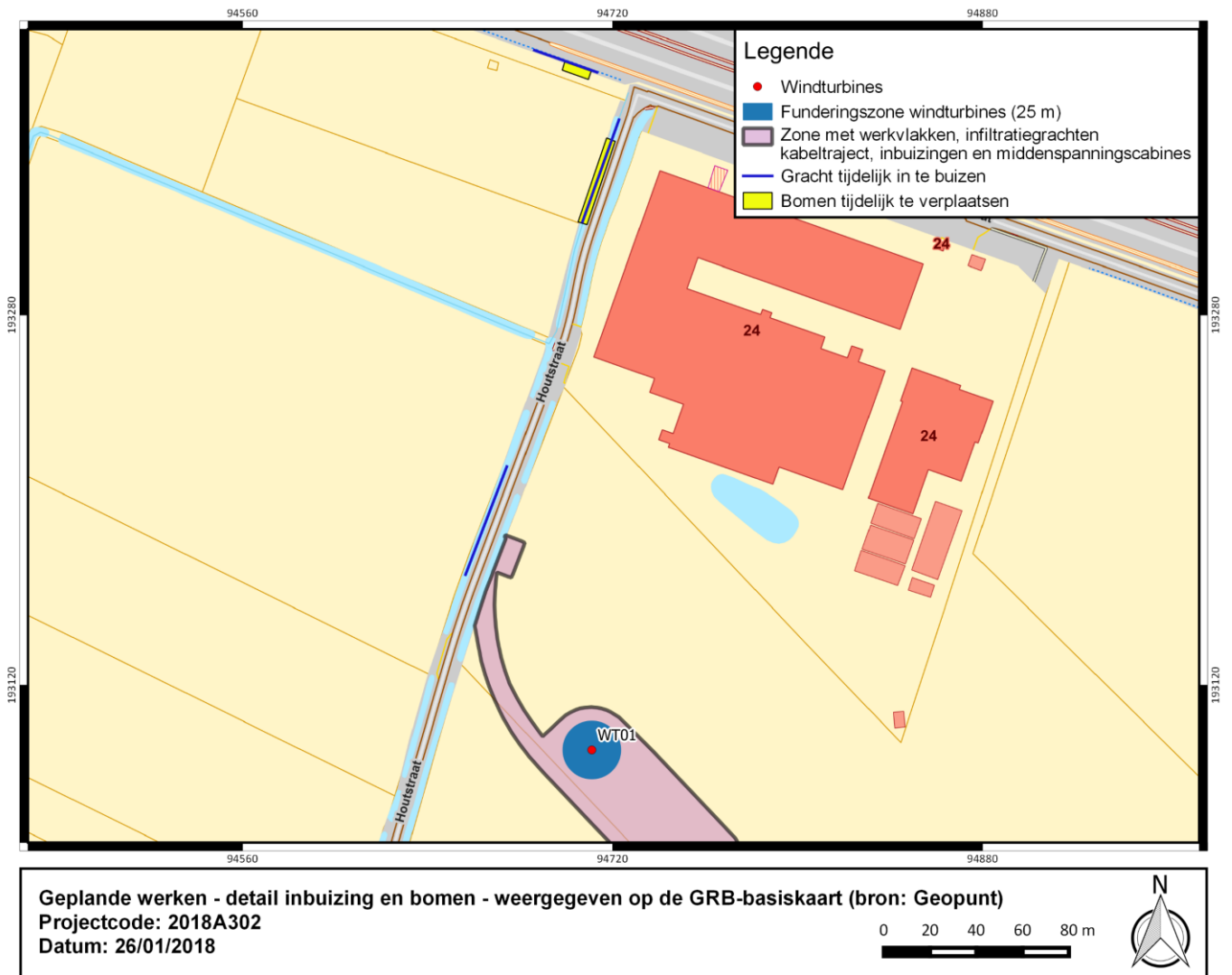
Figuur 2: geplande werken – detail inbuizing en bomen (bron: Geopunt).
