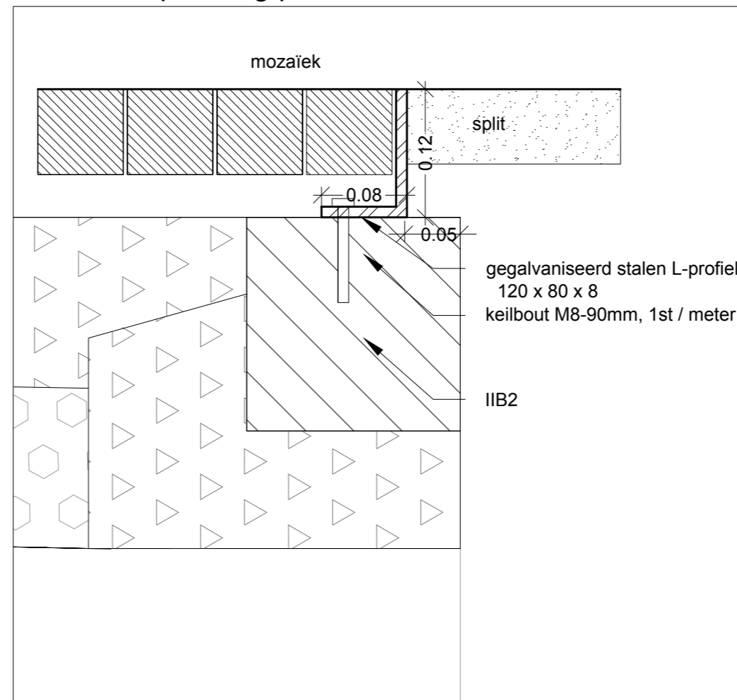
detail B: opsluiting plantvak 1/5
