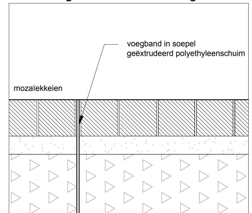
uitzetvoeg elementenverharding 1/5
