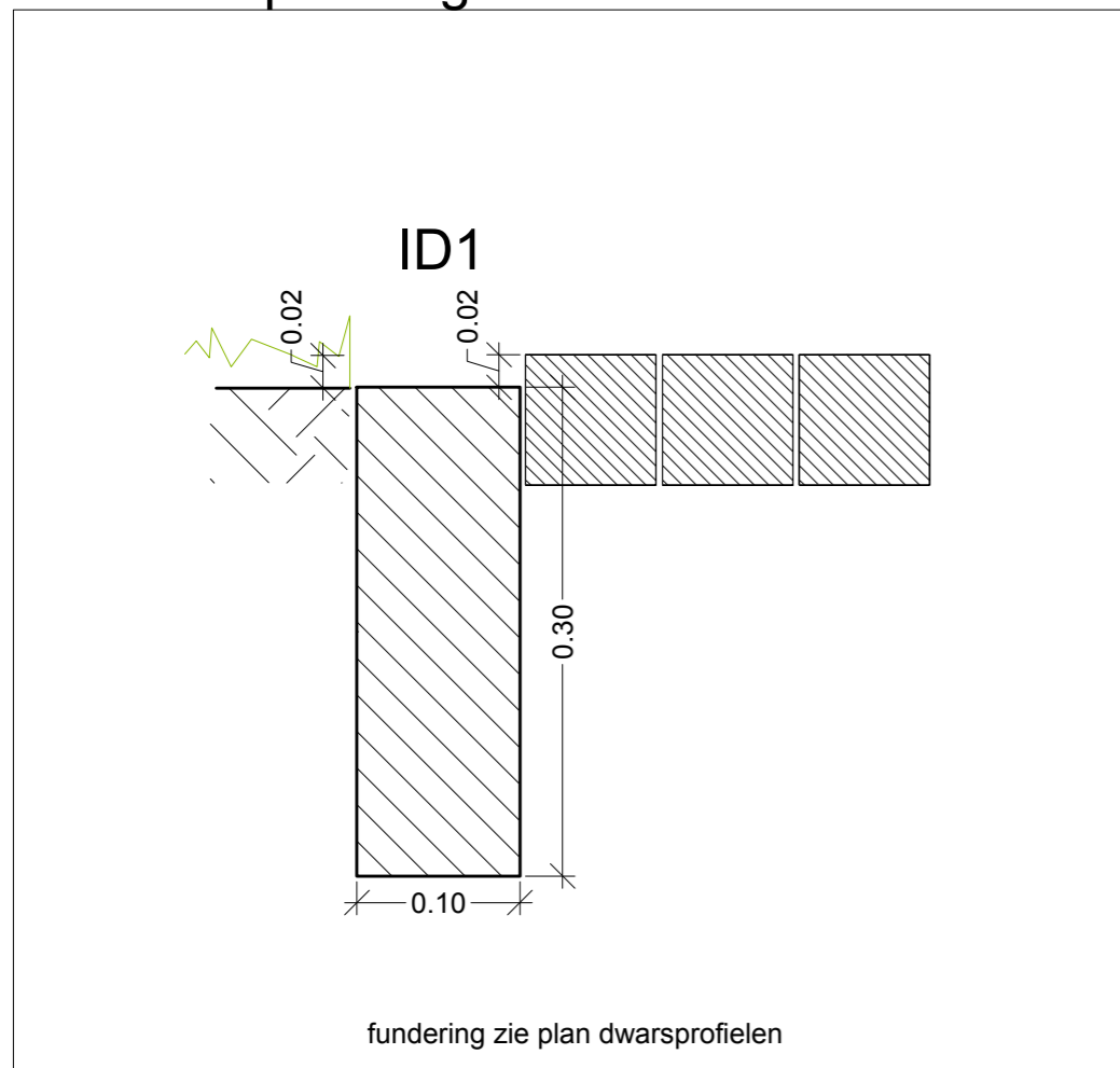
detail A: opsluiting betonband 1/5
