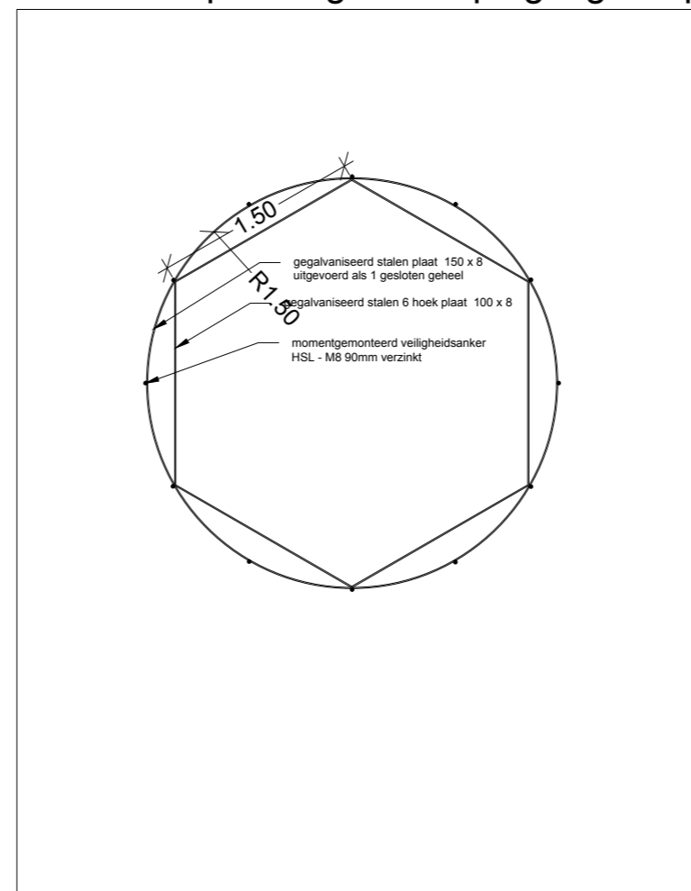
detail C: opsluiting boomspiegel grondplan 1/50
