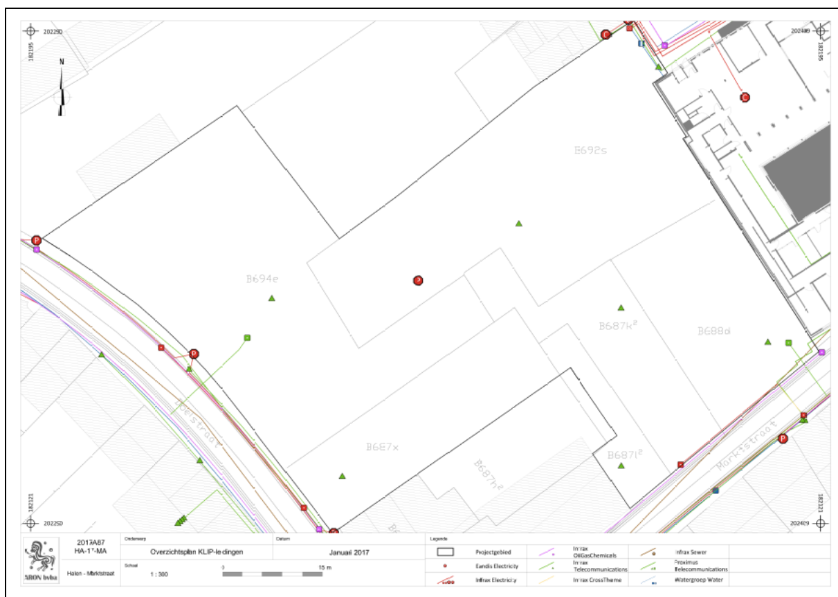
Afb. 39: Overzicht aanwezige nutsleidingen op het onderzoeksterrein (Bron:KLIP, digitaal plan, dd 11/01/2017, aanmaakschaal 1.300, 2017A87)
