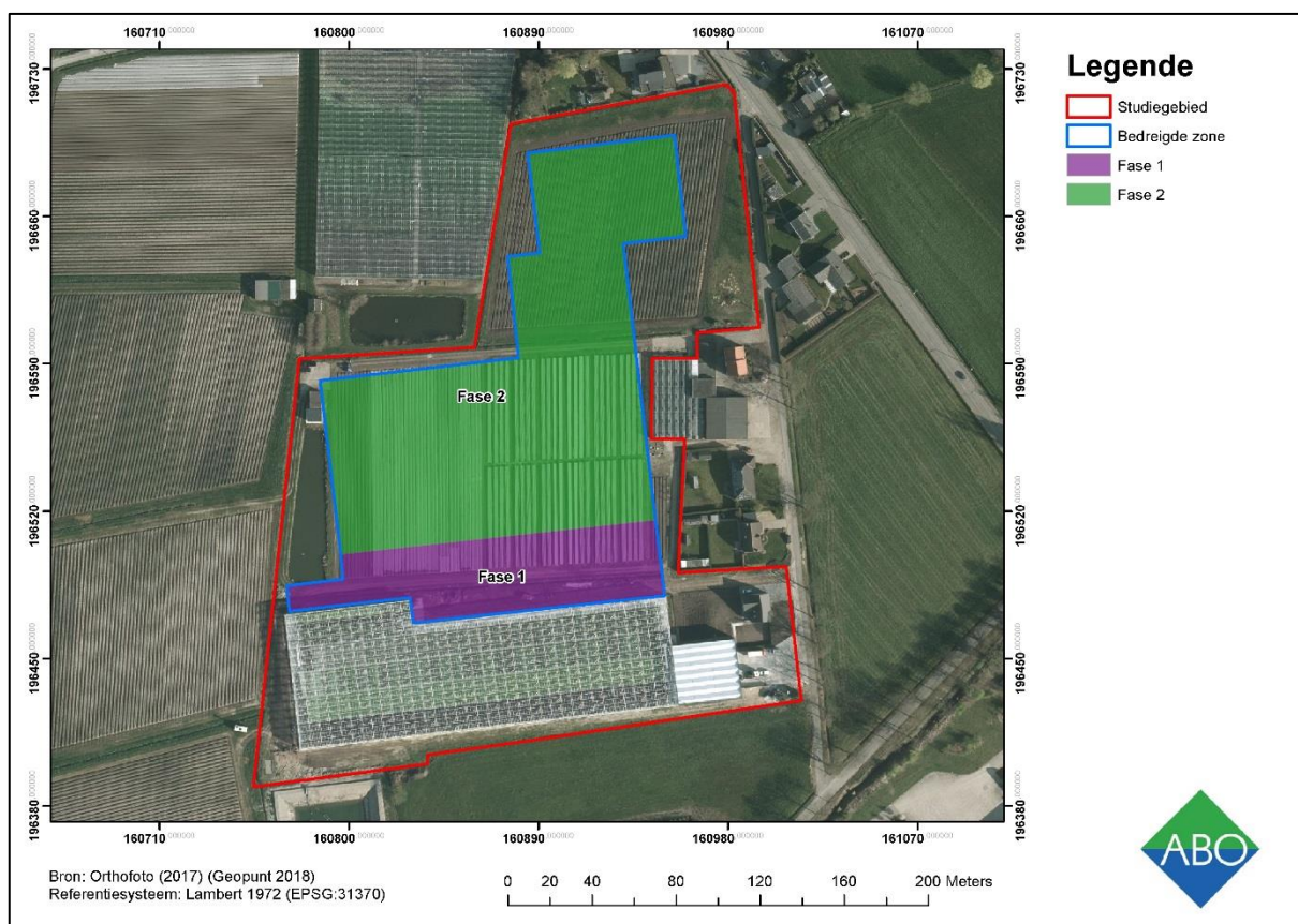
Figuur 3: Schematische weergave van de fasering van de geplande werken weergegeven op een orthofoto (2017) (Geopunt 2018)
