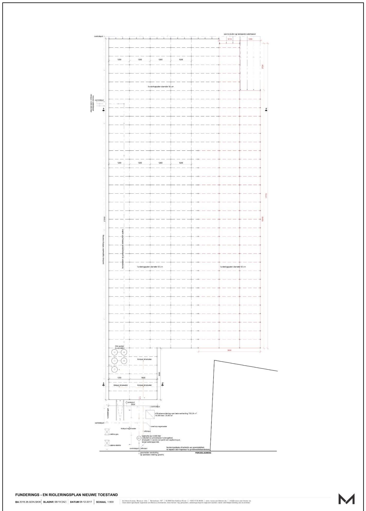
Figuur 5: Funderings- en rioleringsplan van de nieuwe toestand (opdrachtgever 2018)
