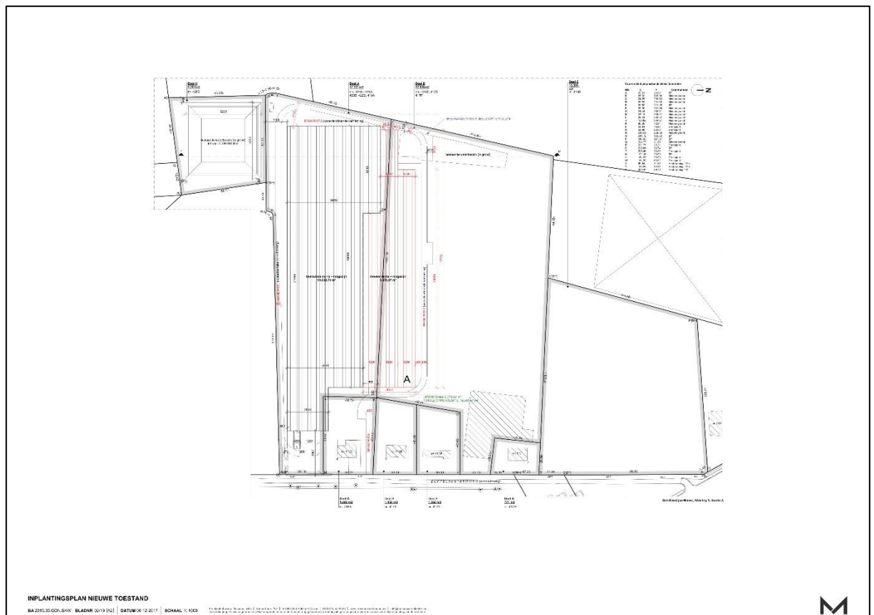
Figuur 4: Bouwplannen van de toekomstige situatie (opdrachtgever 2017)
