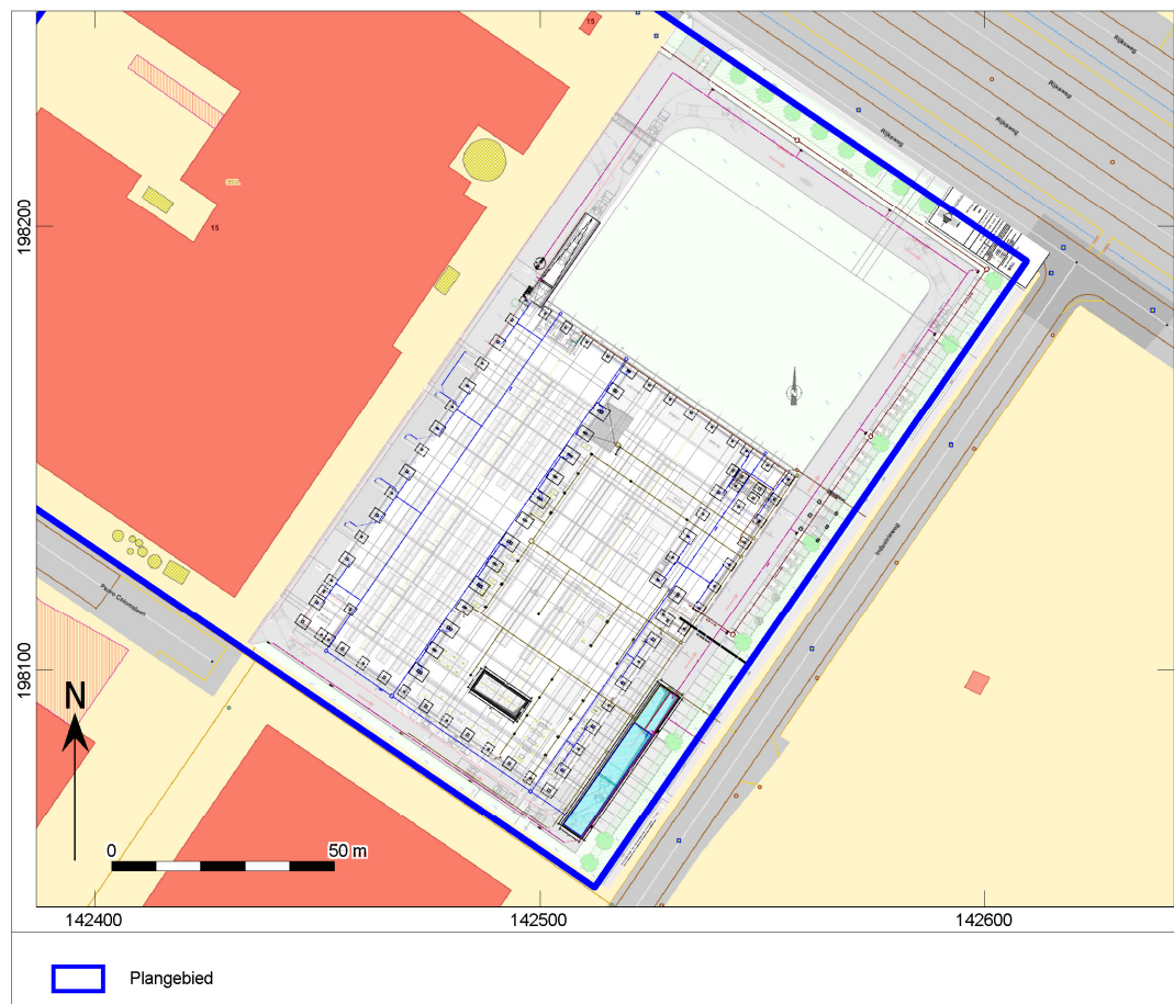
Afb. 5. Rioleringsplan.
