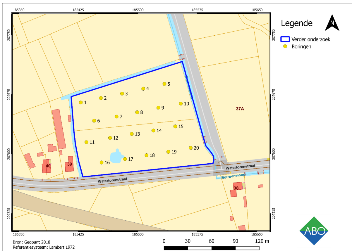
Figuur 4: Landschappelijke boringen in een grid van 25 op 30 meter. (Schaal 1:1500).
