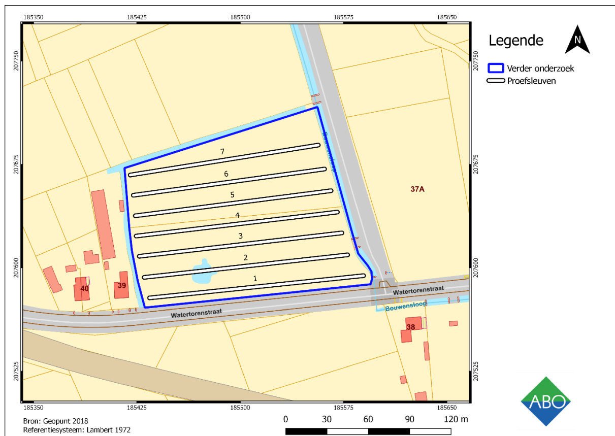
Figuur 5: Plan voor de optionele proefsleuven op het onderzoeksgebied. (Schaal 1:1500).
