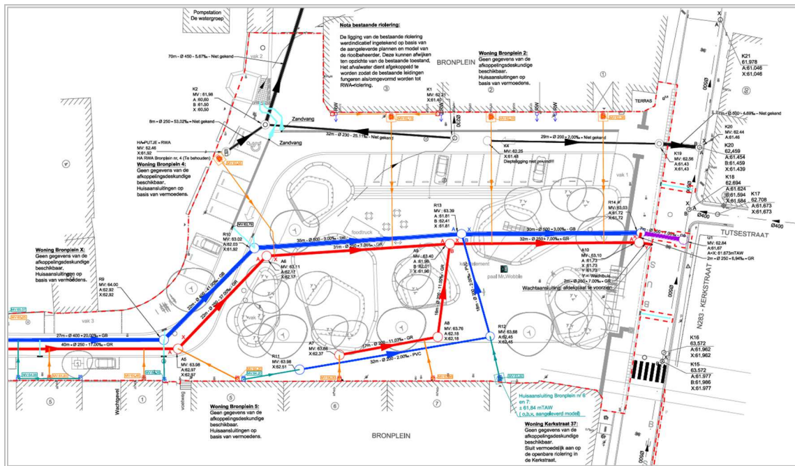
Figuur 4: Rioleringsplan, detail Bronplein (D+A Consult, 2018)
