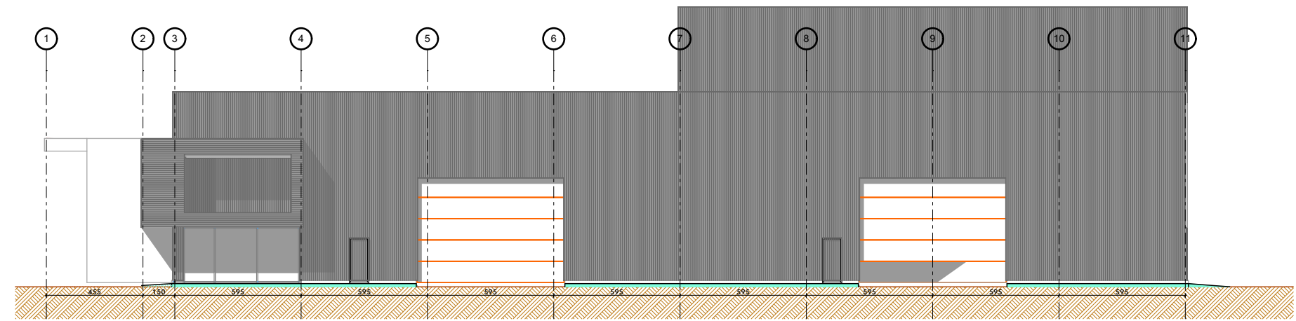
Voorgevel
