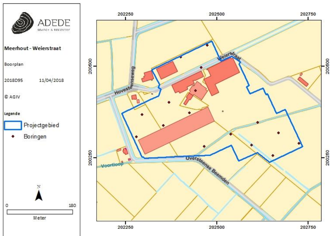
Figuur 2. Boorplan.
