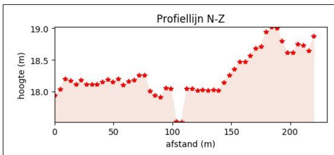
Figuur 17: Hoogteprofiel noord-zuid (Geopunt 2018)
