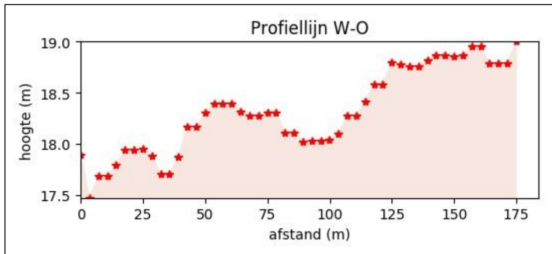
Figuur 18: Hoogteprofiel west-oost (Geopunt 2018)
