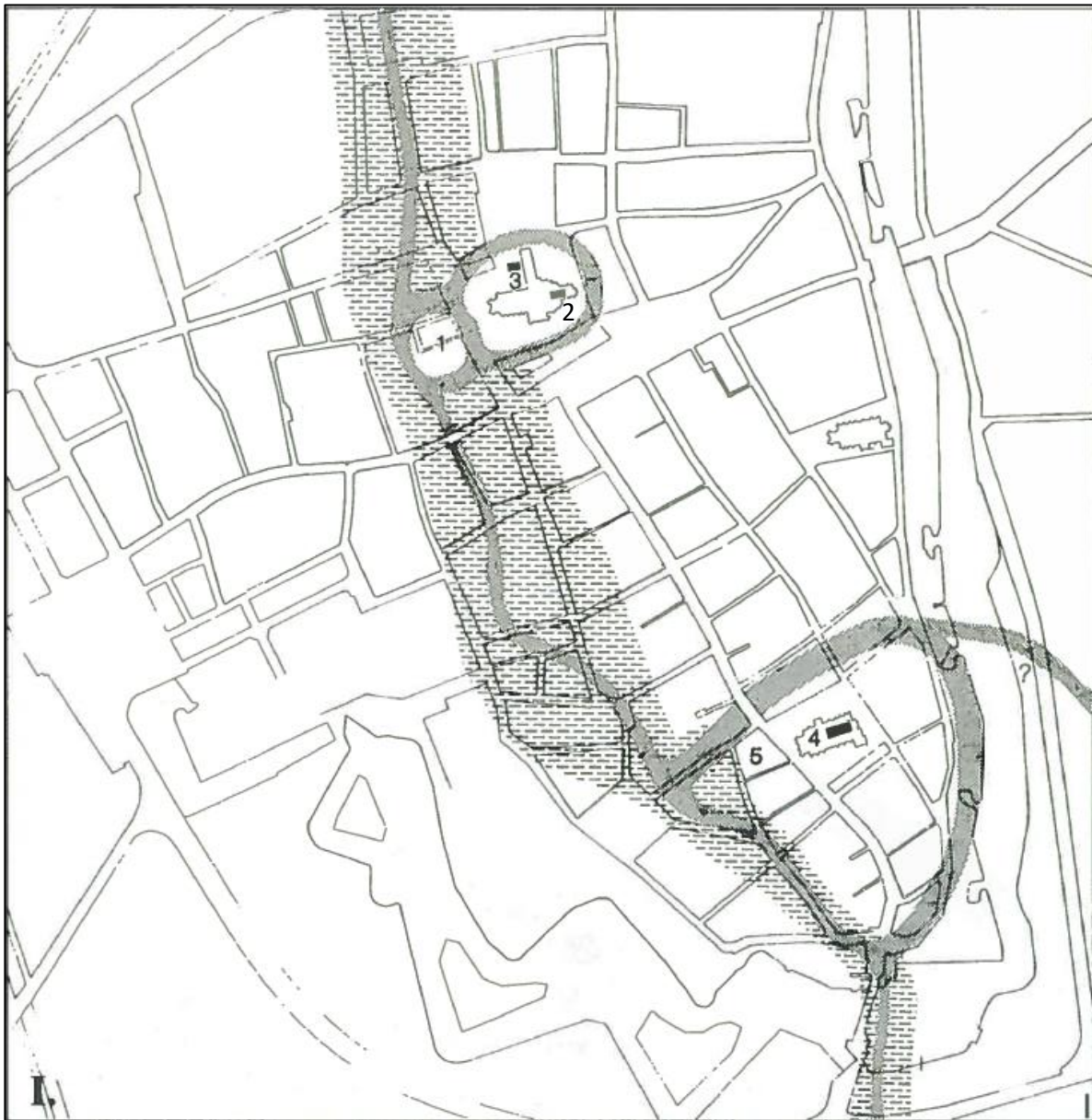
Figuur 26: oudste kernen van leper. Legende: 1. Motteheuvel 2. Castrale kapel Sint-Martinus 3. Grafelijke spijker voor graanopslag 4. Sint-Pieterskerk 5. Marktplaats. Het raster geeft de zone van het alluvium aan. (Termote J., 1990)
