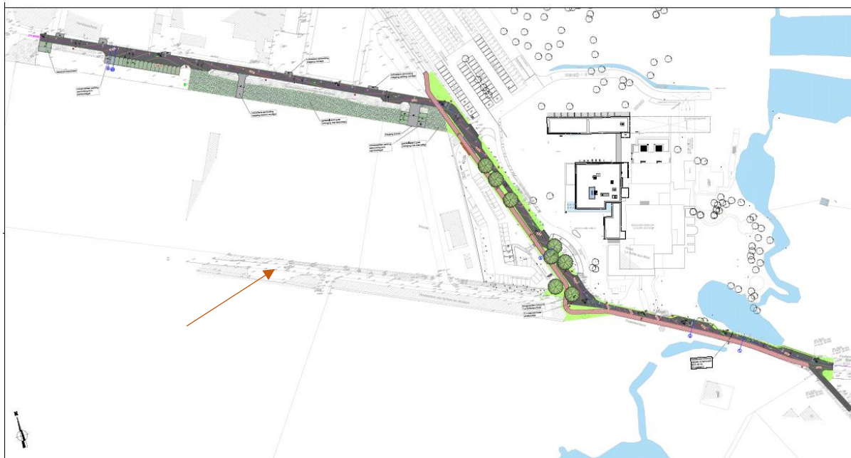
Afb. 3: Ontwerpplan met dwarsprofielen (Bron: Geotec, digitaal plan, dd. 31/05/2018, aanmaakschaal 1.500, 2017G23)
