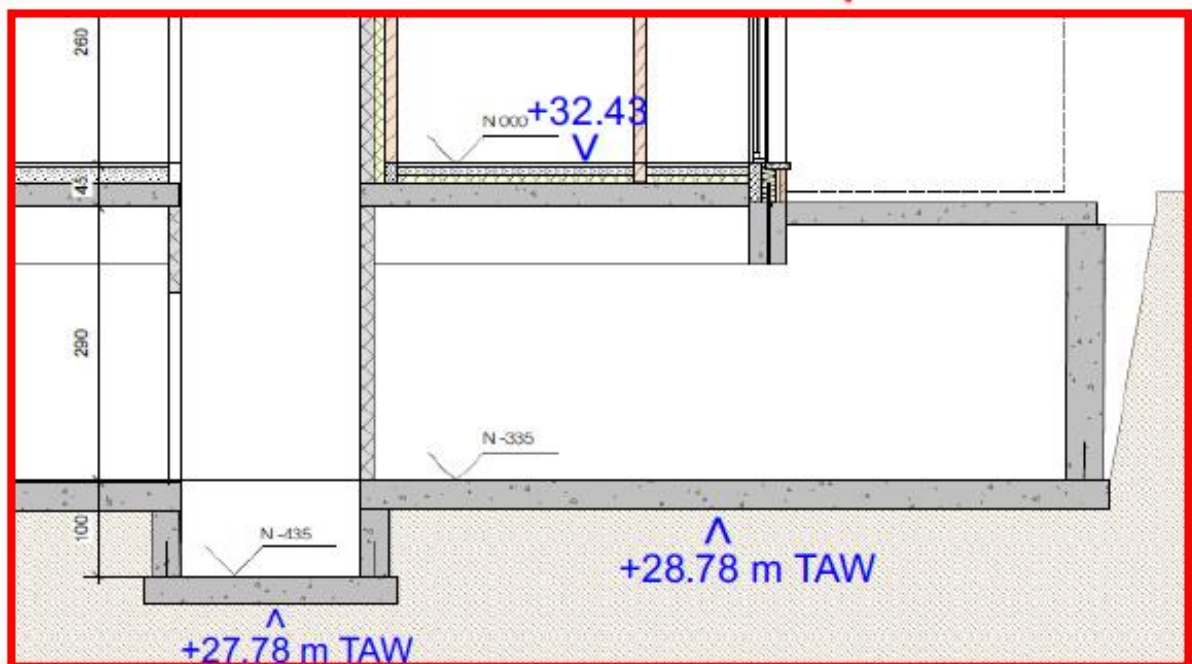
Fig. 8: detail uit doorsnede B' - B van de te bouwen kelder © arch. Vranken
