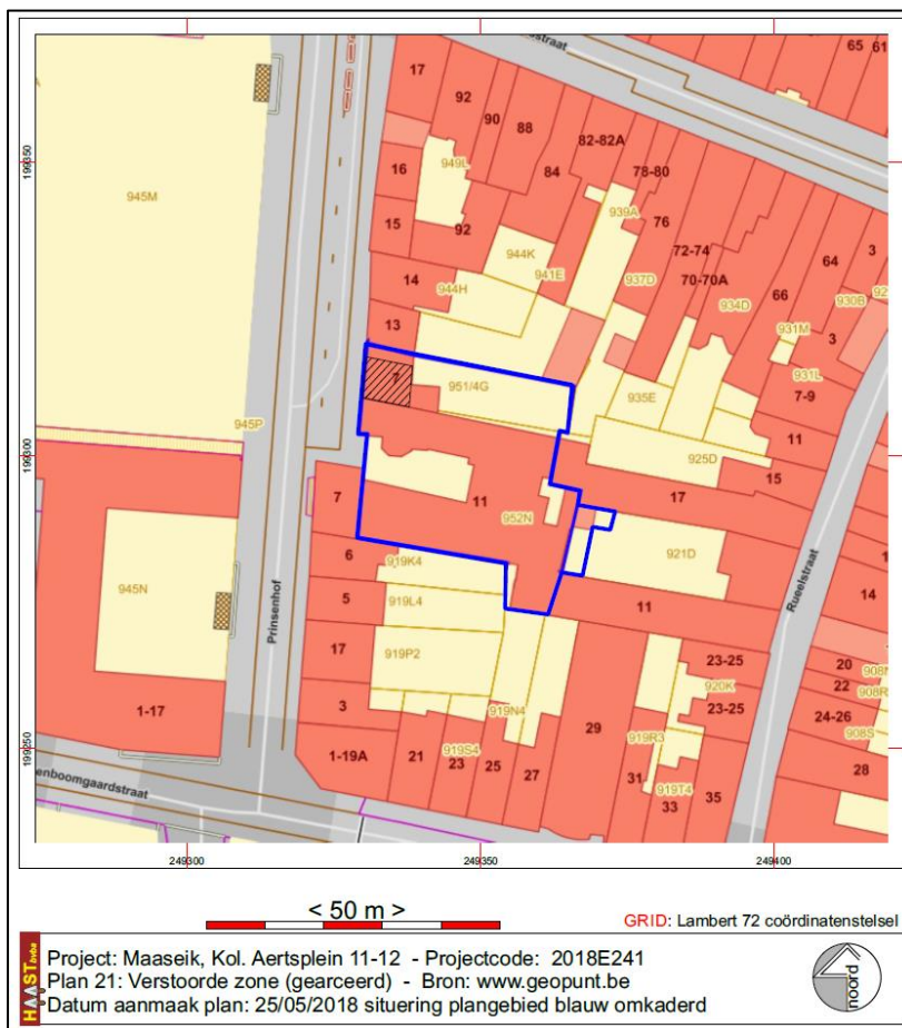
Fig. 37: verstoorde zones
