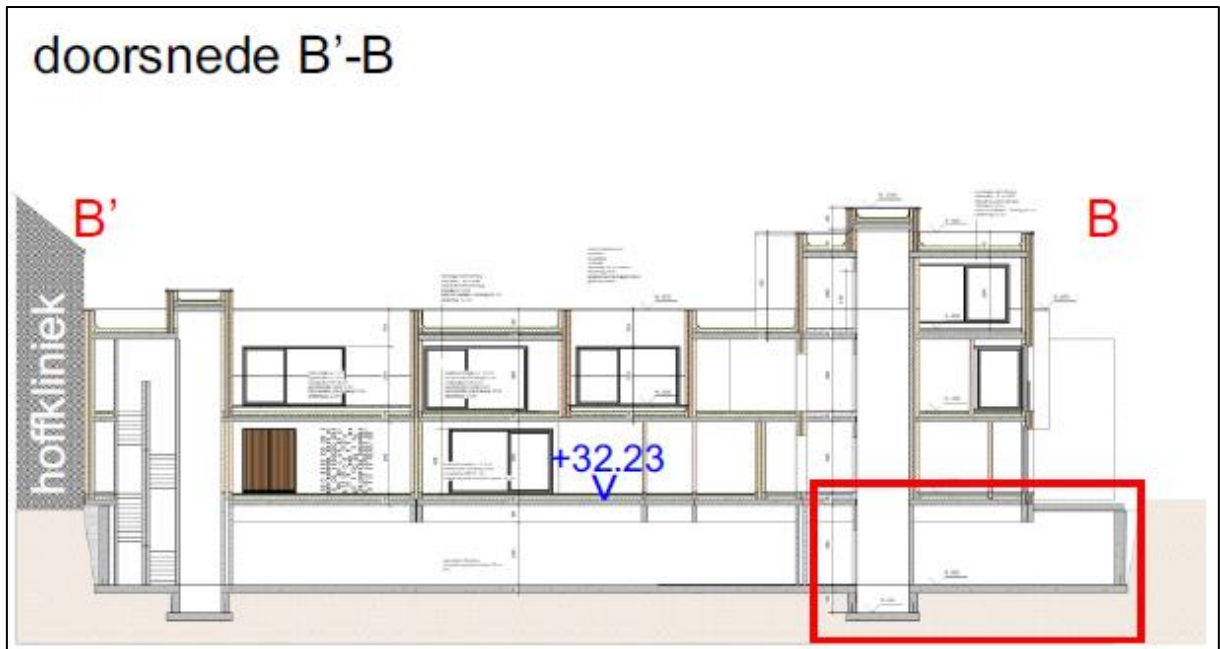
Fig. 7: doorsnede B' - B van de te bouwen kelder © arch. Vranken
