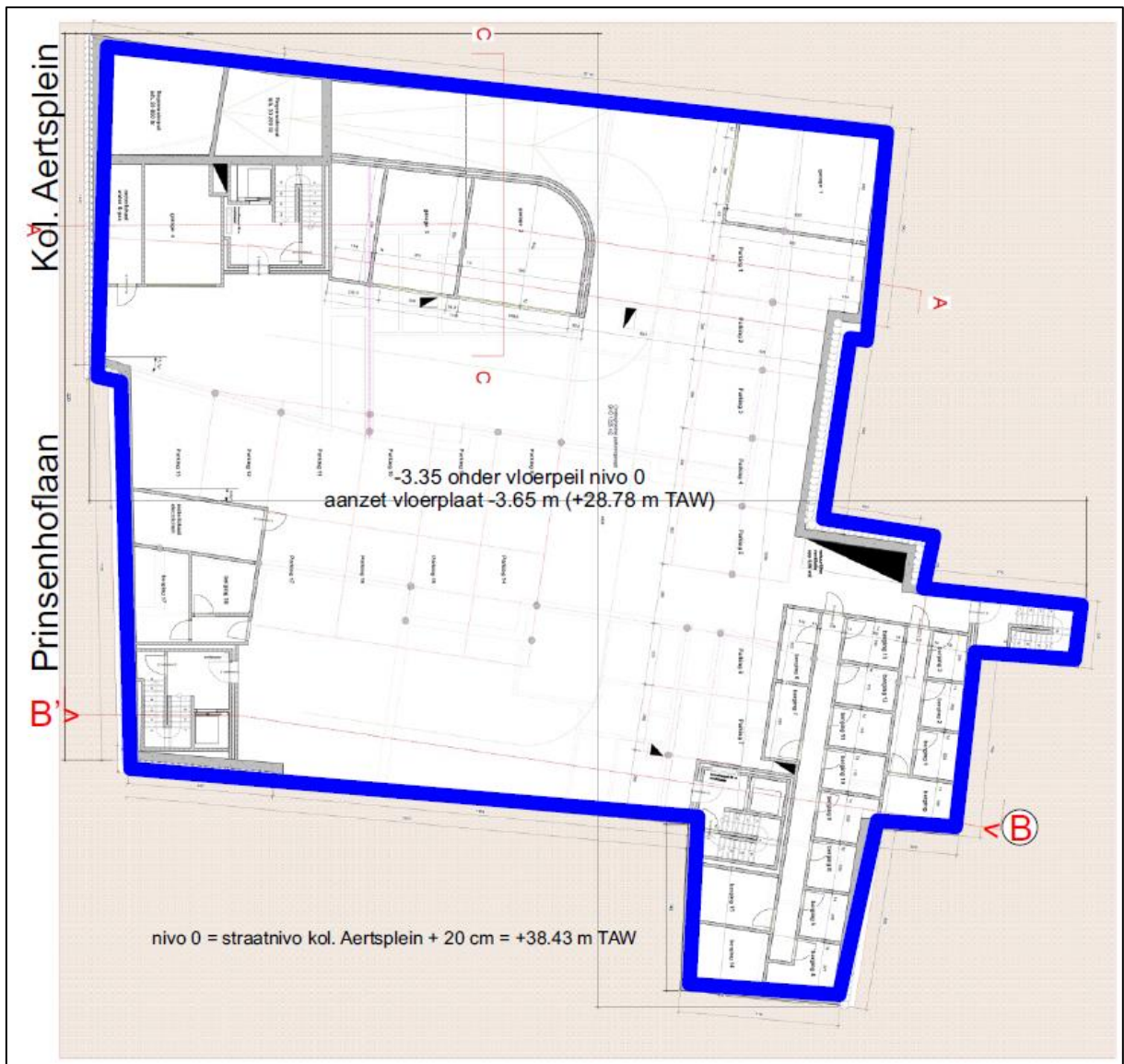
Fig. 6: kelderplan van de nieuwbouw © arch. Vranken
