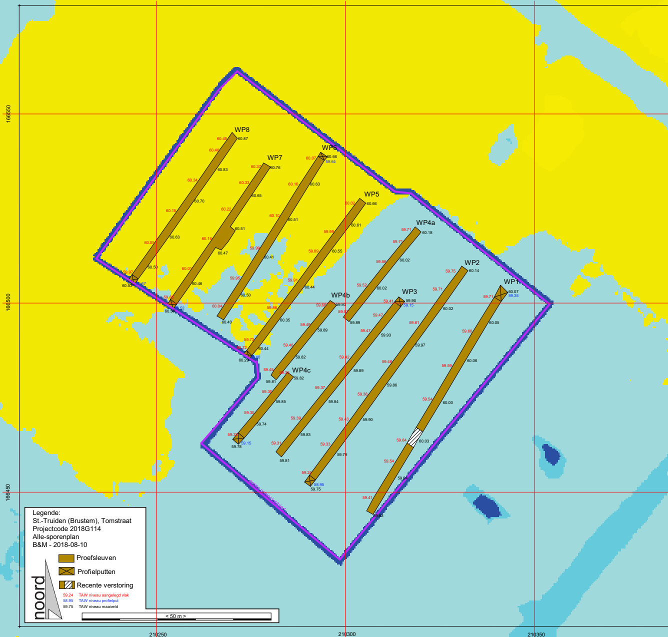
2018G114 - Projectie alle-sporenplan op het geïnterpoleerd Digitaal Hoogtemodel, terreinmodel - 1 m
