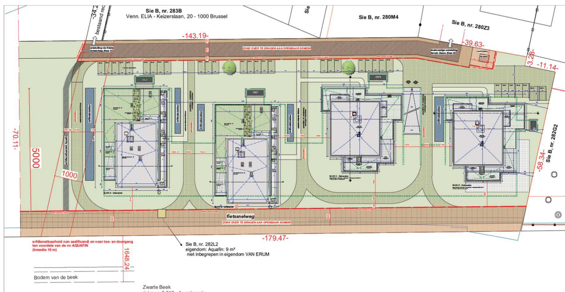
Figuur 7: Grondplan van toekomstige inplanting (d&d architecten, 2018)
