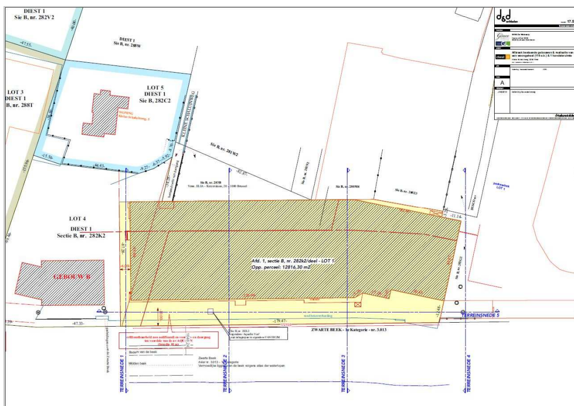
Figuur 5: Grondplan van de huidige bebouwing (D&d architecten, 2018)
