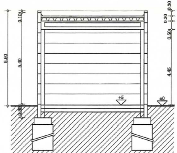
snede cc
