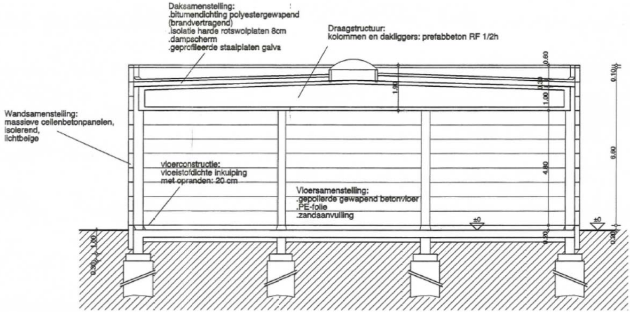
snede bb fundering op putten; diepte volgens sonderingsverslag
