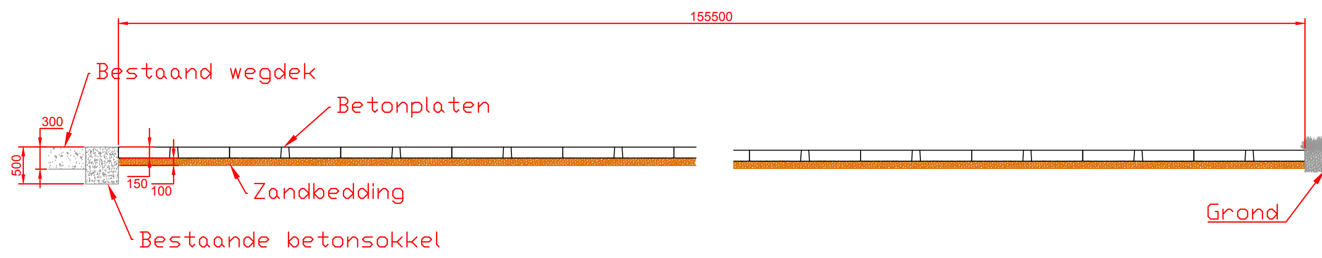
TERREINPROFIEL C-C
