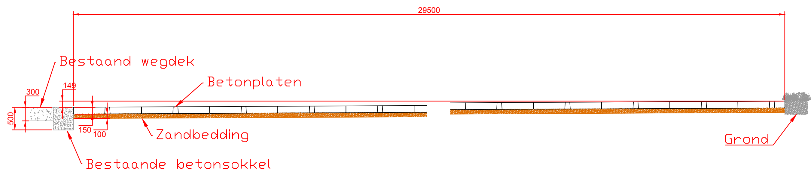
TERREINPROFIEL B-B
