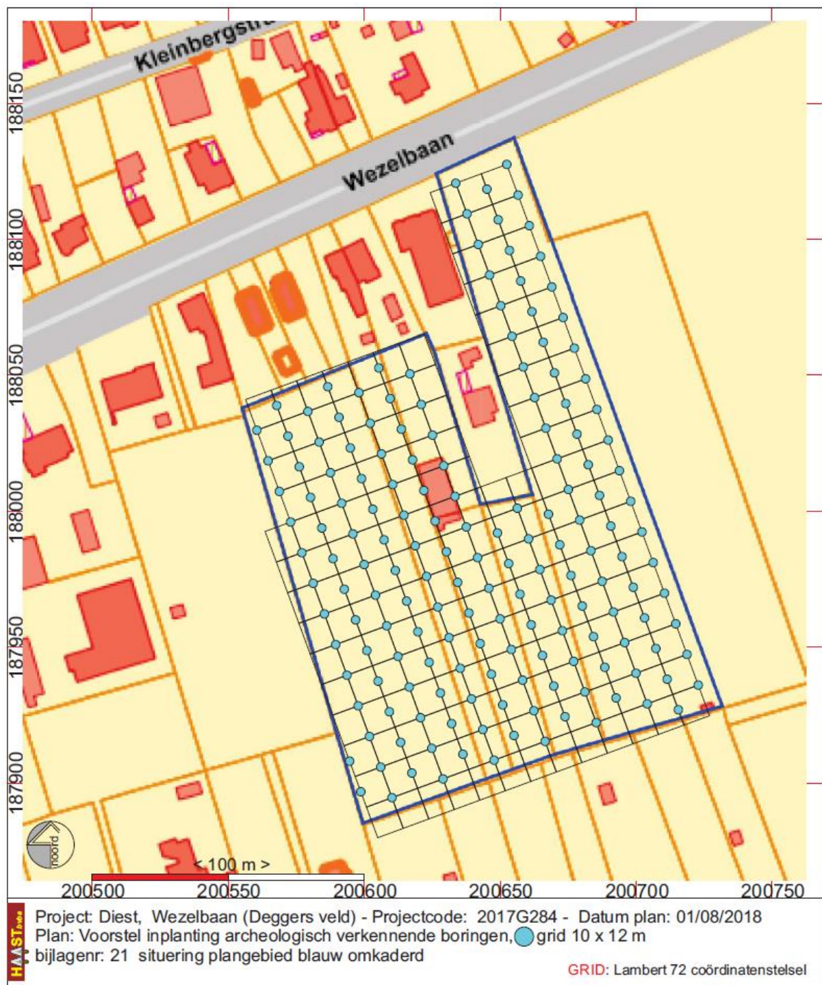
Fig. 6: Voorstel inplanting boorpunten verkennend archeologisch booronderzoek ervan uitgaande dat er door het landschappelijk bodemonderzoek geen zones uitgesloten kunnen worden voor aanwezigheid van steentijdsites
