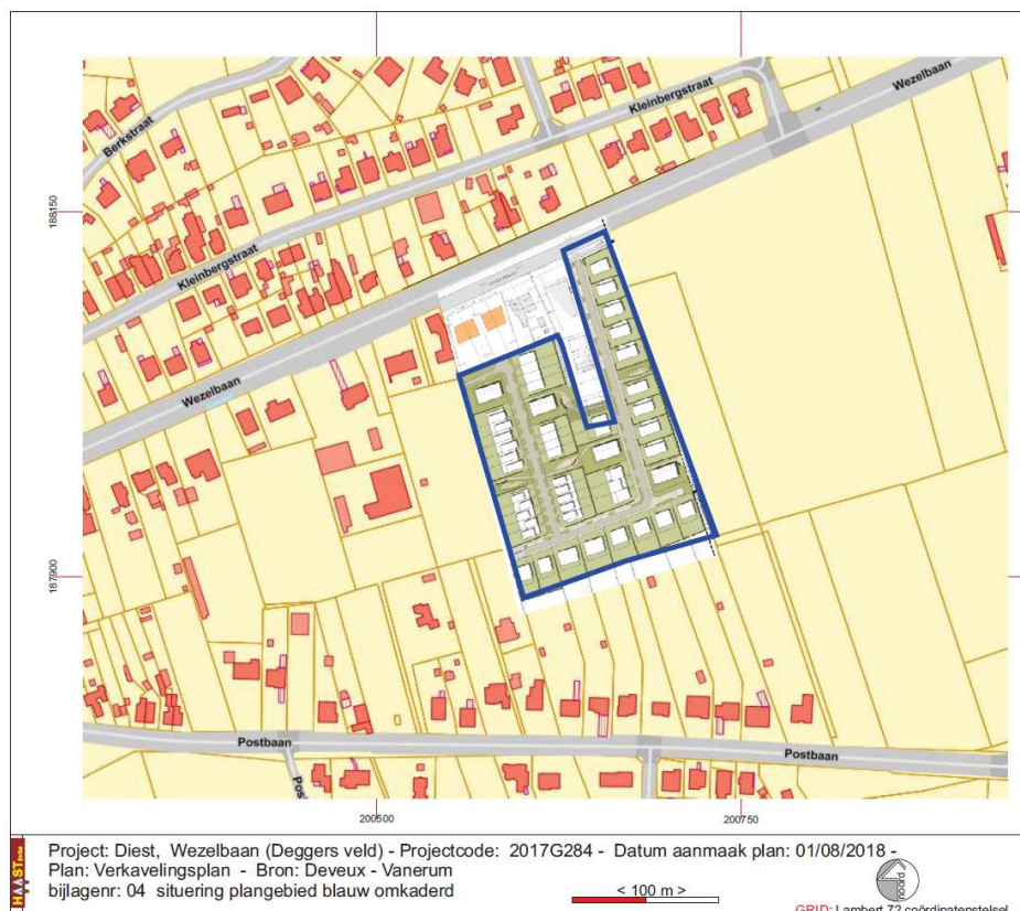
Fig. 3: Gegeoreferentieerd verkavelingsplan. © Deveux – Vanerum
