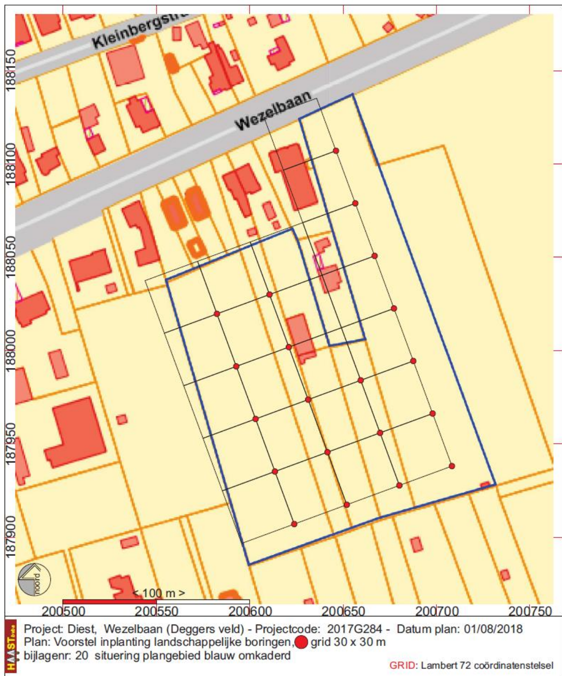
Fig. 5: Voorstel inplanting landschappelijke boorpunten
