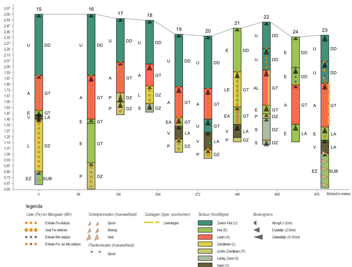
figuur 42: Verkleinde weergave van het originele profiel van de boorresultaten in zone 3 van het onderzoeksgebied (zie bijlage 6). ©RAAP België
