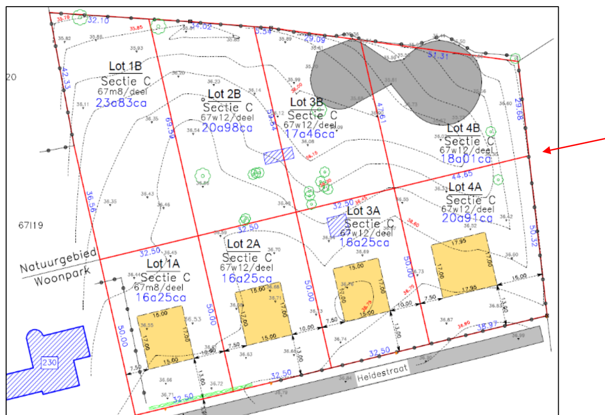
Fig. 3: Opsplitsing natuurgebied – woonpark zoals aangeduid op het verkavelingsplan © aaro-topo.
