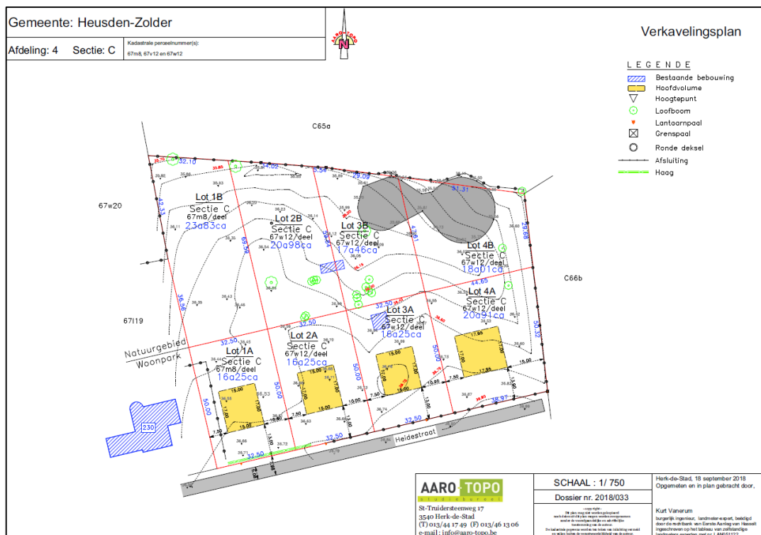
Fig. 5: verkavelingsplan zoals aangereikt © Aaro-topo
