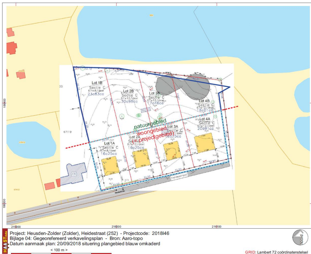
Fig. 4: Gegeoreferend verkavelingsplan. © Aaro-topo
