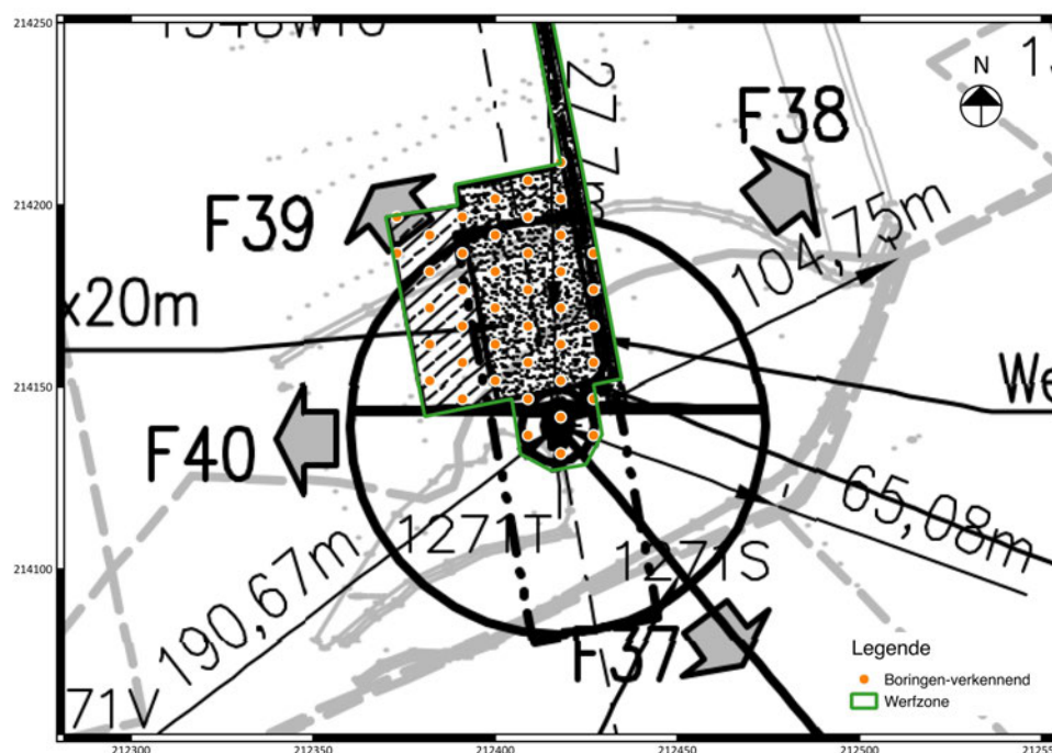
Fig. 3.2: Voorstel tot inplanting van verkennende boringen in een grid van 12 x 10 meter ter hoogte van de windturbine 7 en de werfzone 66 . De inplanting is vergelijkbaar voor windturbine 4.
