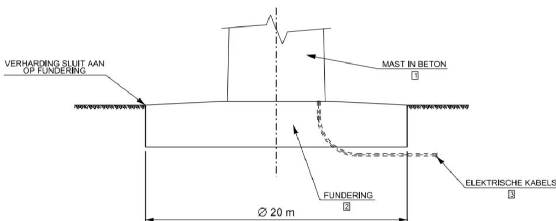
Figuur 7: Doorsnede fundering windturbine (bron: opdrachtgever).
