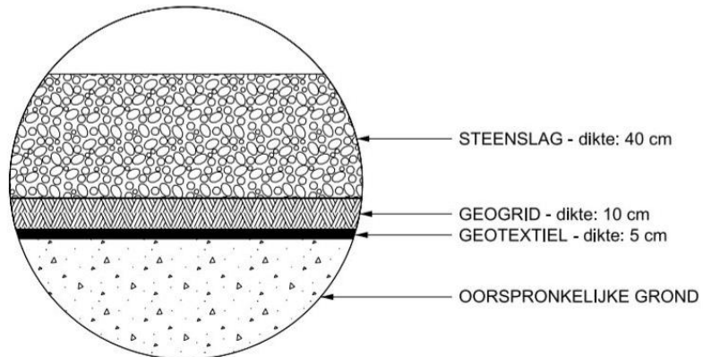
Figuur 8: Doorsnede toegangsweg (bron: opdrachtgever).
