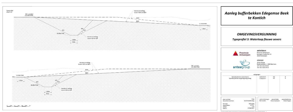
Figuur 2. Dwarsdoorsnedes van de geplande bodemingrepen: aanleg van een waterloop met flauwe oevers (inclusief poelen) ter hoogte van het bufferbekken (bron: Provincie Antwerpen, Dienst Integraal Waterbeleid)
