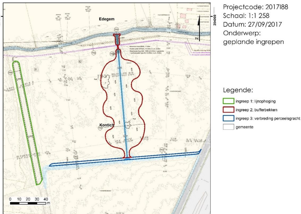
Figuur 1. Overzicht van de locatie en aard van de geplande bodemingrepen (bron: Provincie Antwerpen, Dienst Integraal Waterbeleid).
