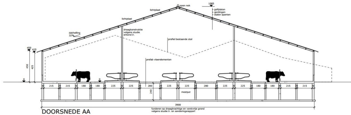
Figuur 6: Doorsnede van de toekomstige stal 7
