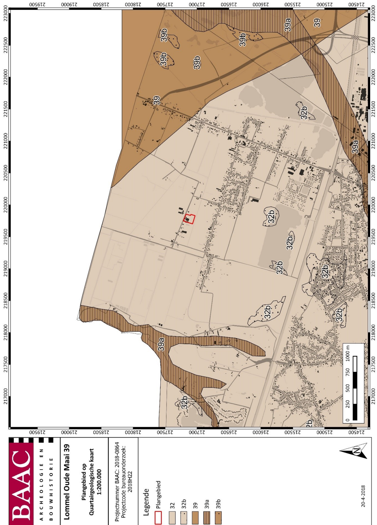
Figuur 13: Plangebied op de Quartaairgeologische kaart 1:200.000 25
