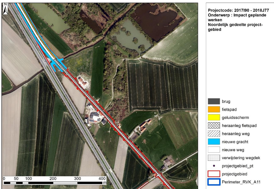
Figuur 4 : Geplande werken in het zuiden van het projectgebied
