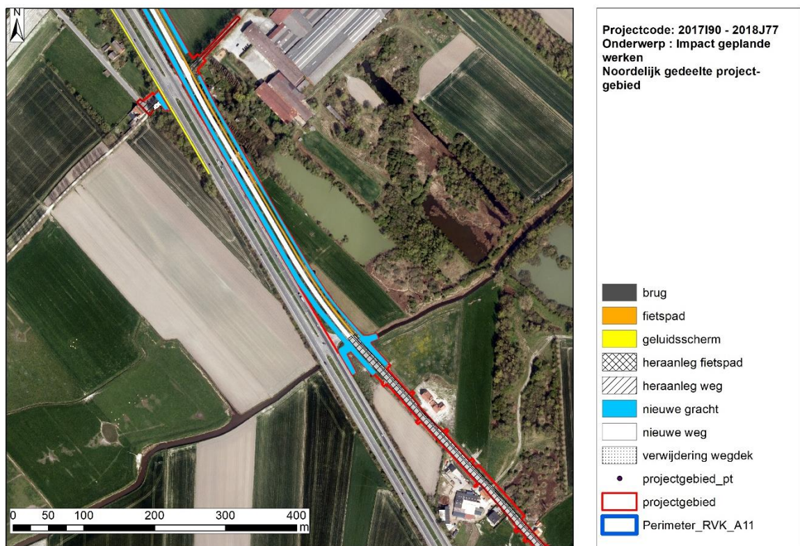
Figuur 3 : Geplande werken ten zuiden van de Damse Vaart
