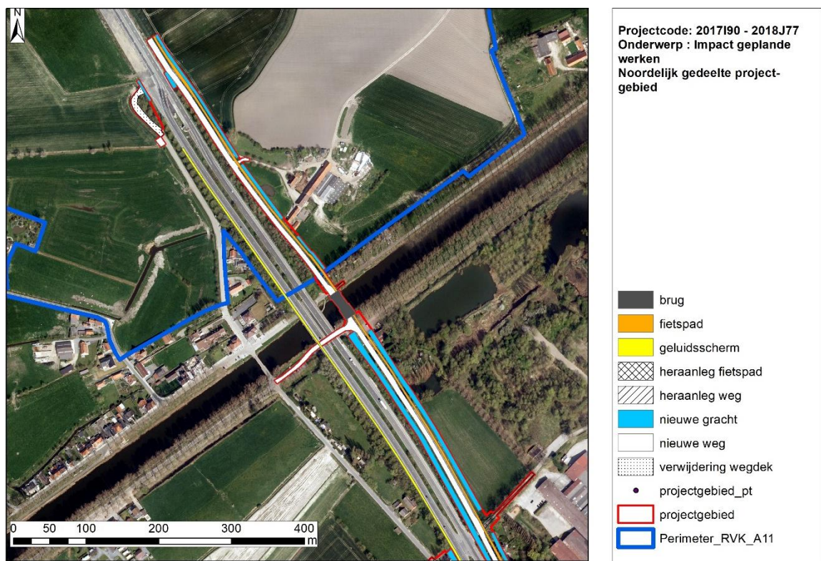
Figuur 2 : Geplande werken in het noorden van het projectgebied
