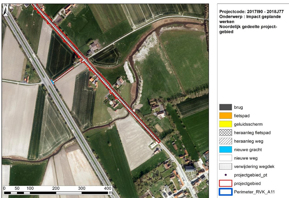
Figuur 5 : Geplande werken in het zuiden van het projectgebied
