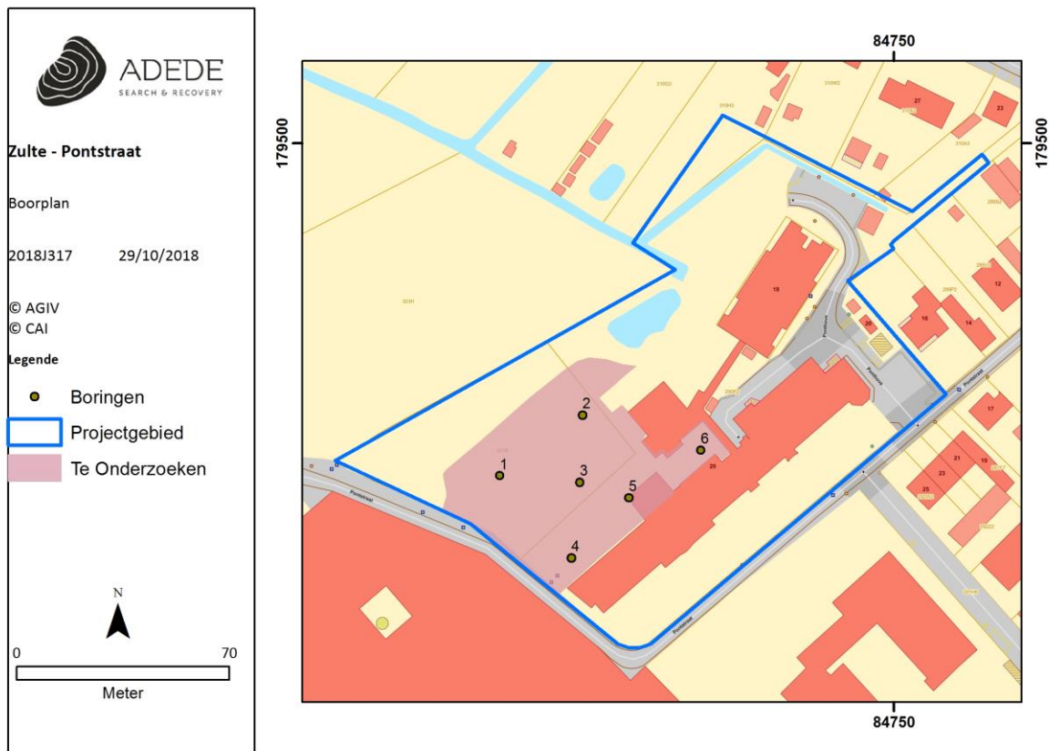
Figuur 2. Boorplan.
