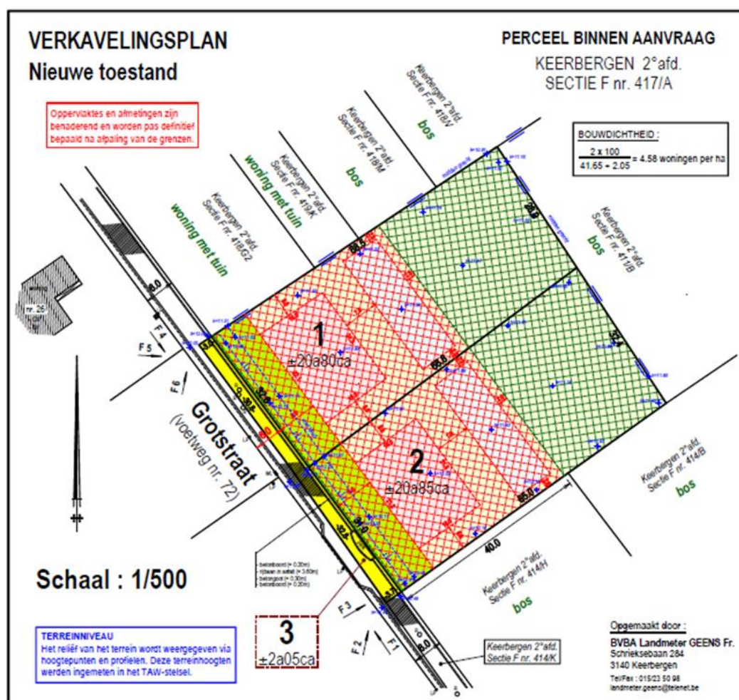
Figuur 2: Ontwerpplannen voor de verkavelingsaanvraag (Fr. Geens, 2017)
