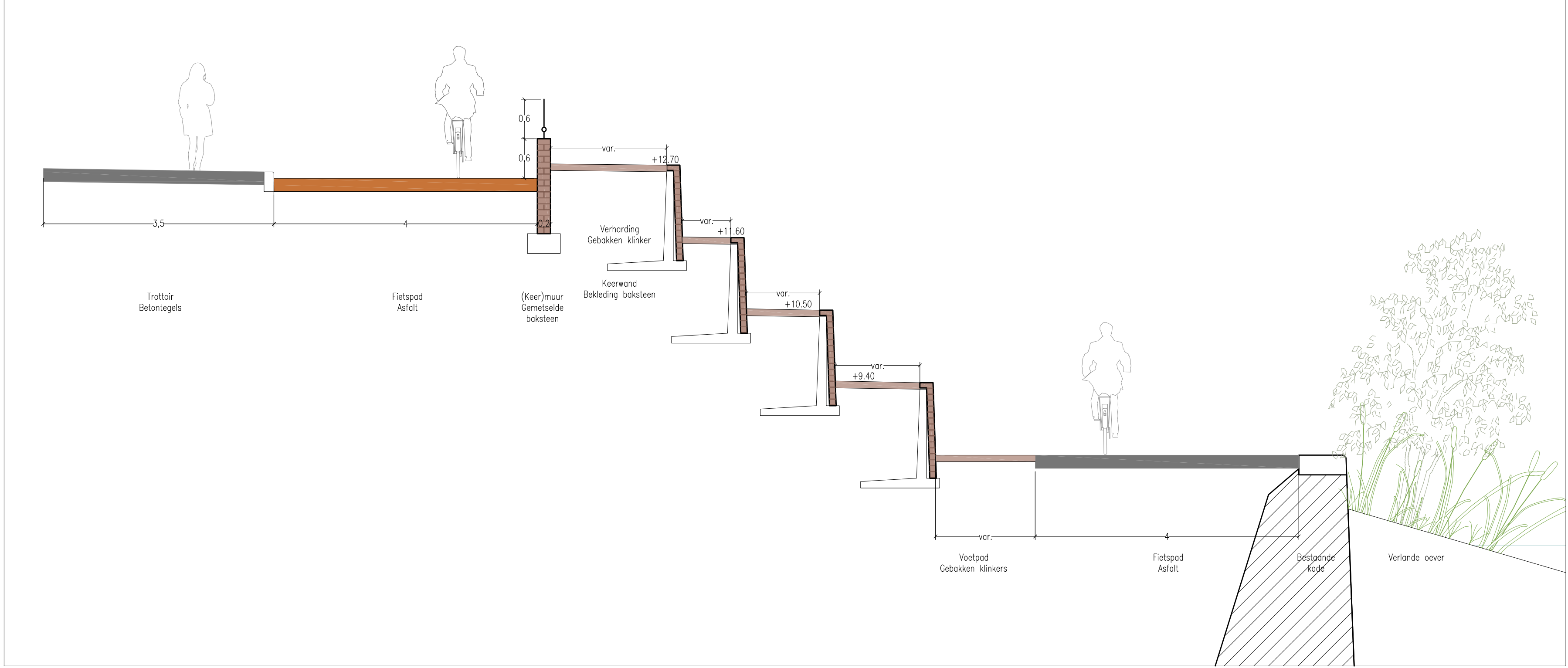
KOH: principesnif 01 1:50
