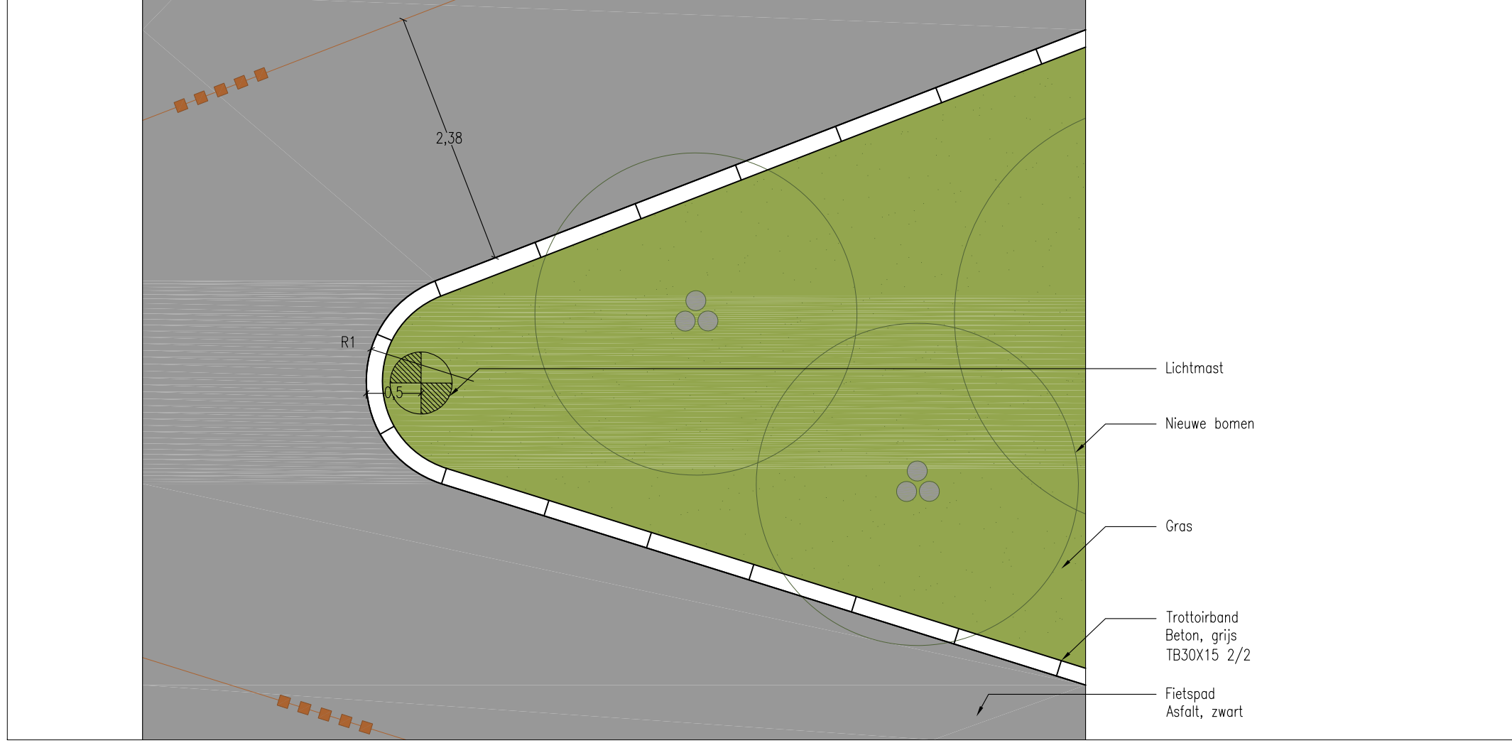
KOH: principedetail 02 1:50
