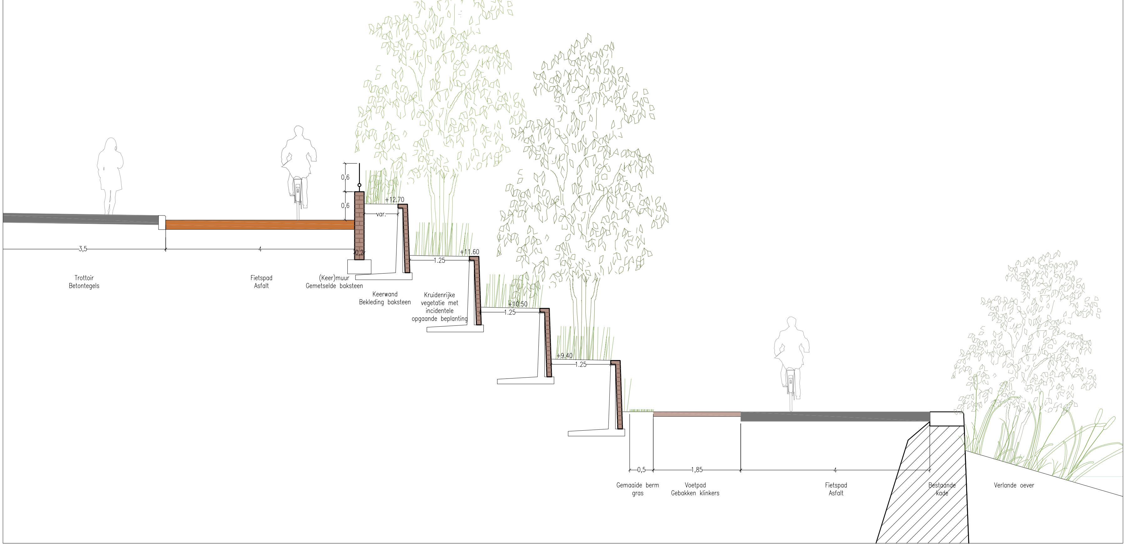
KOH: principesnif 02 1:50
