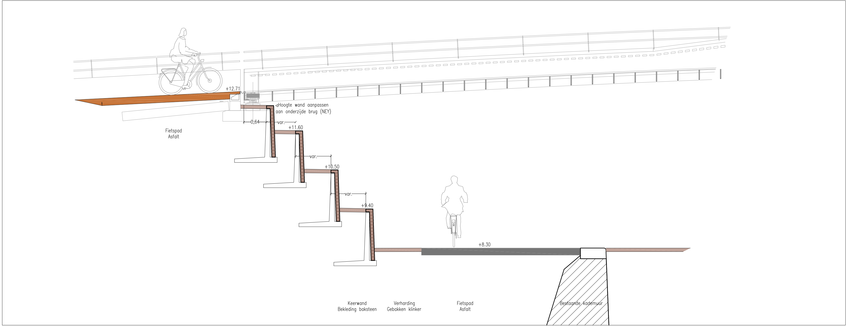
KOH: principesnif 03 1:50
