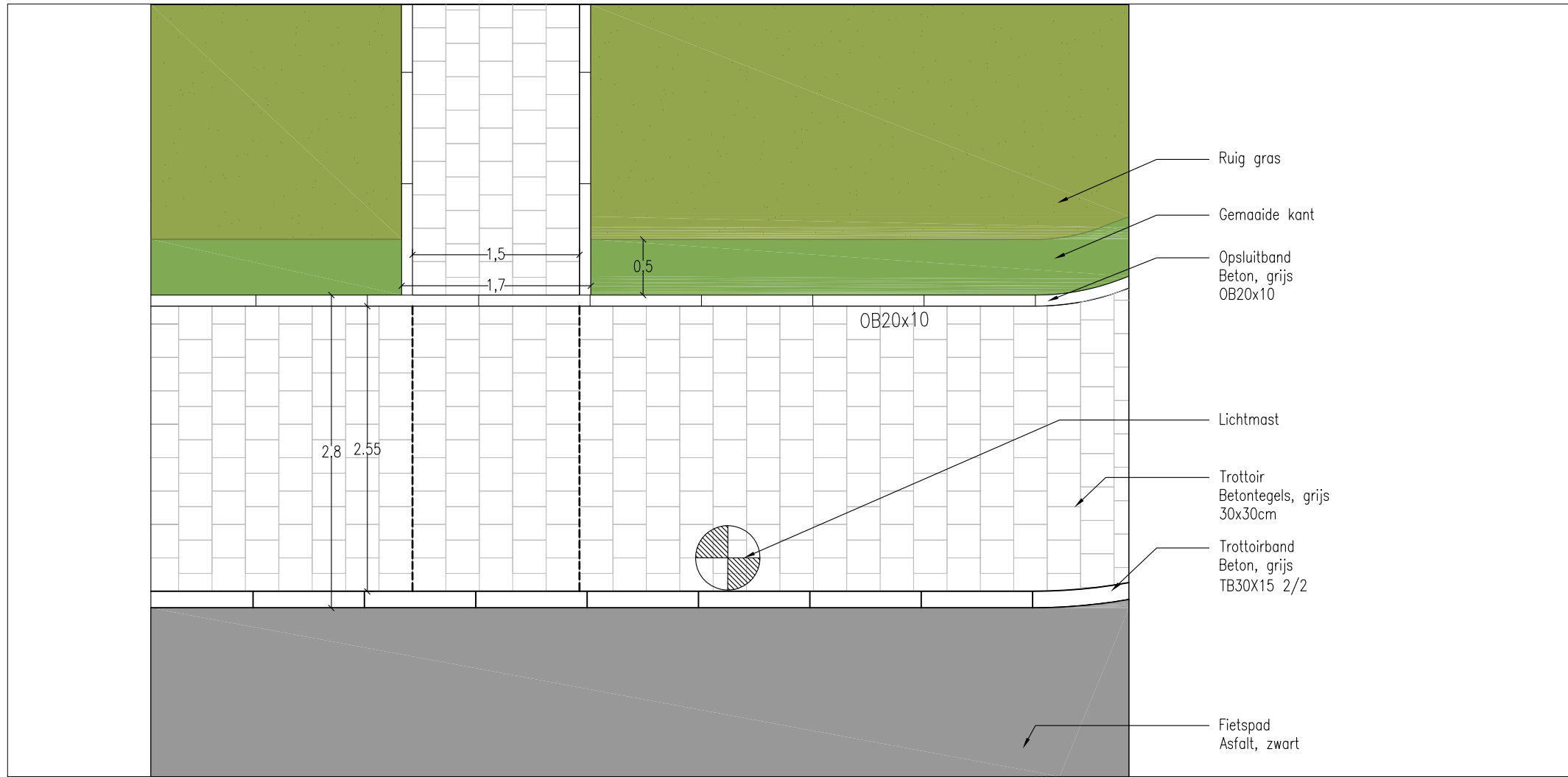
KOH: principedetail 03 1:50
