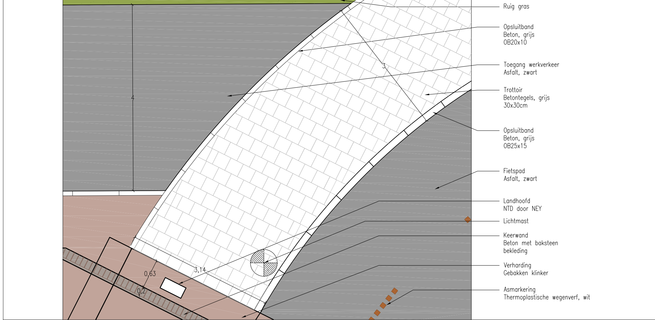
KOH: principedetail 04 1:50
