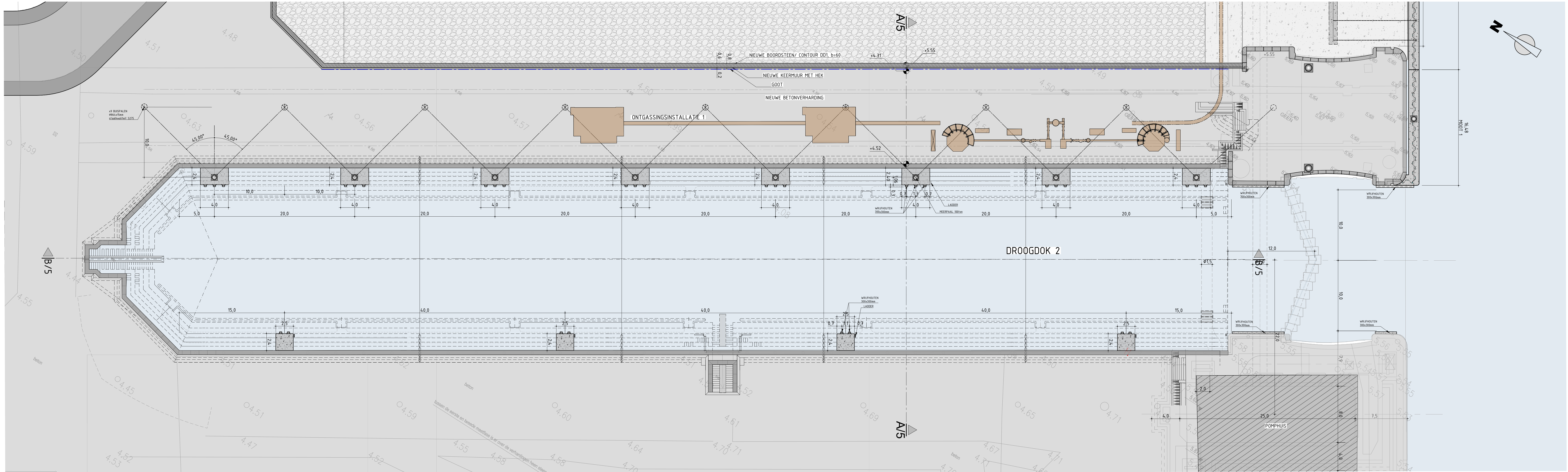
GRONDPLAN_DD2_NIEUWE TOESTAND SCHAAL: 1/200 0 5 10 15 20m
