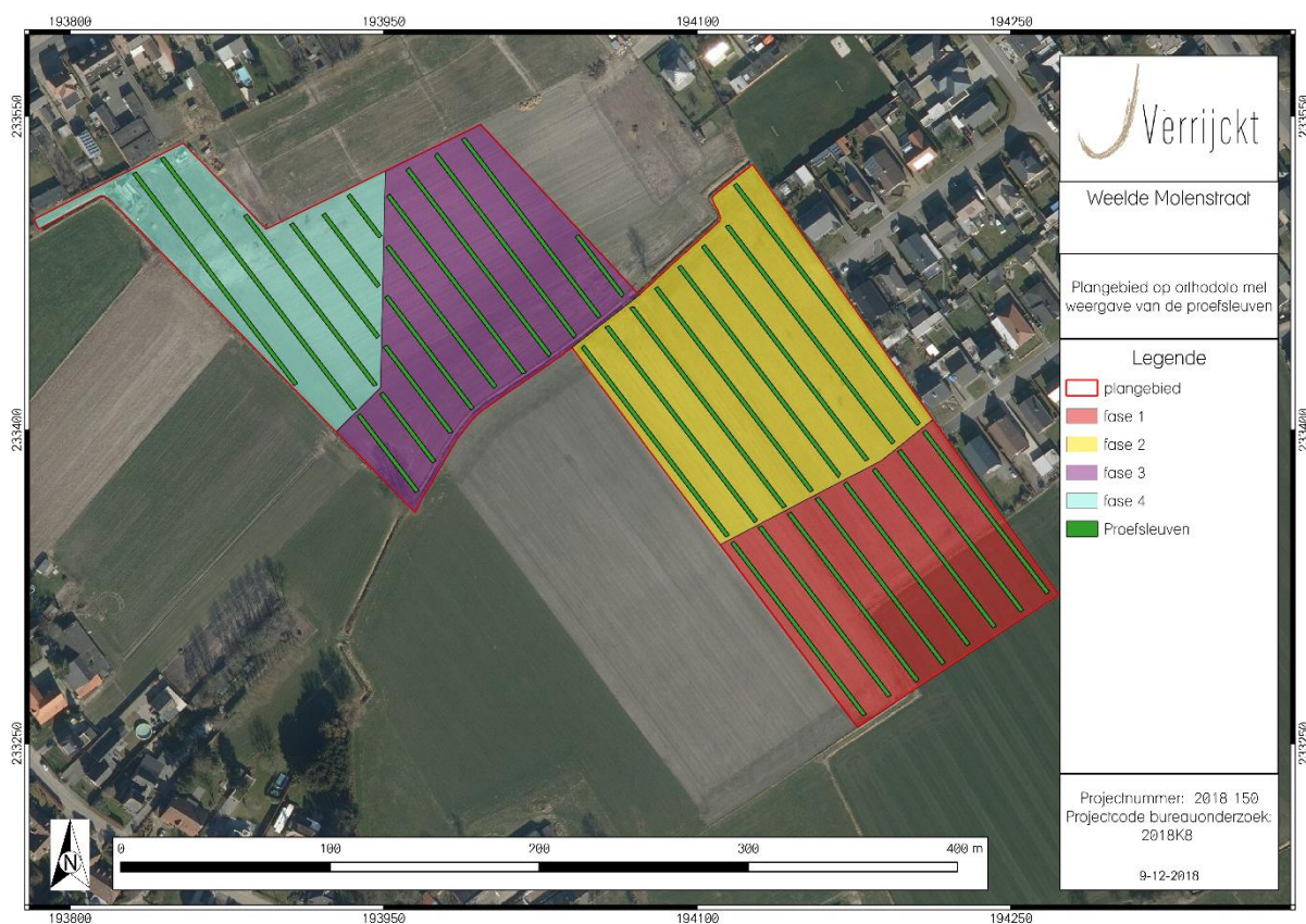
Figuur 3: Sleuvenplan
